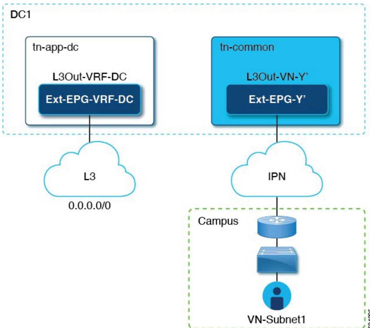
図 5 L3Out 接続
