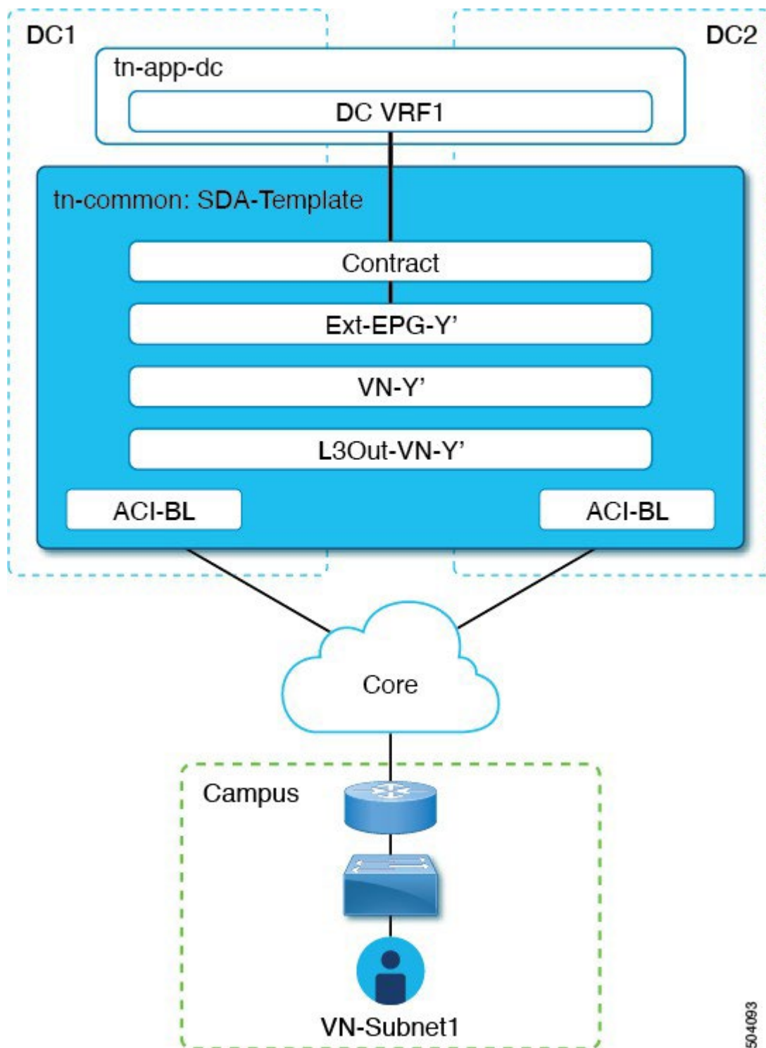
図 3. VRF へのマッピング
