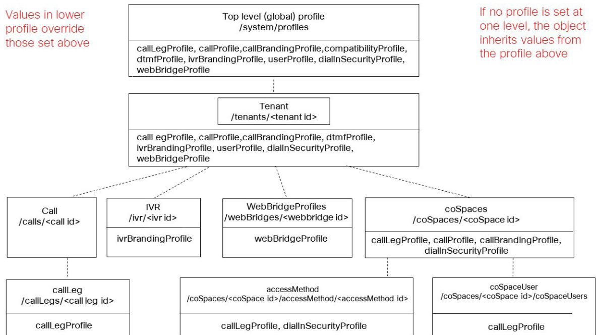
図 6 : テナント使用時のプロファイルでの値の継承
