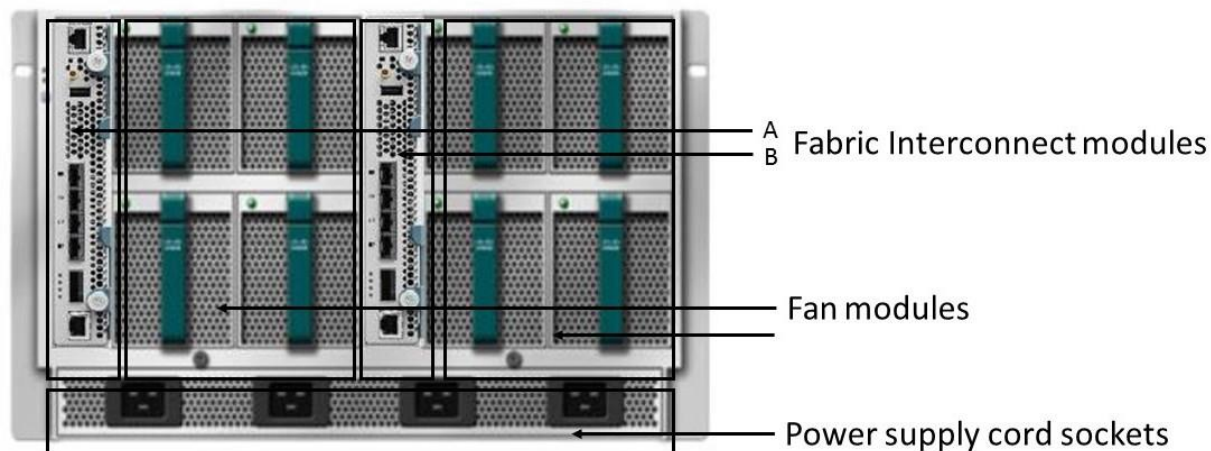
図 2：ユニットの背面にはファブリック インターコネクト モジュール、8 個のファンモジュール、4 個の電源コードソケットが示されています
