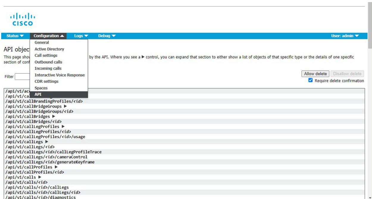
図 2：ミーMeeting Server Web インターフェイス経由で Call Bridge API にアクセスする
