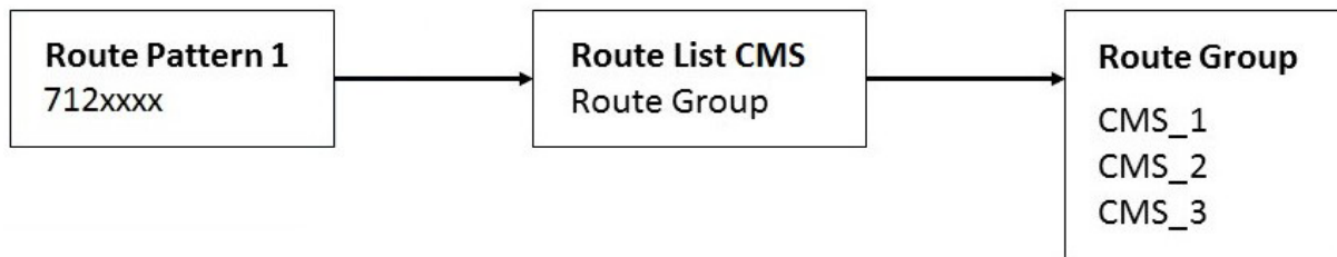
図 3: 通話を正しいロケーションに転送する
