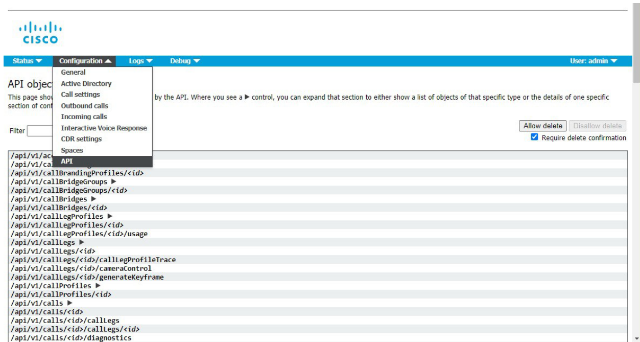
図 2 : Meeting Server のウェブ管理インターフェイス経由で API にアクセスする
