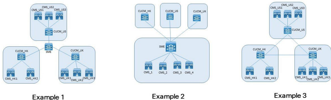
図 4：着信呼び出しをロードバランシングするための 3 つの導入例
