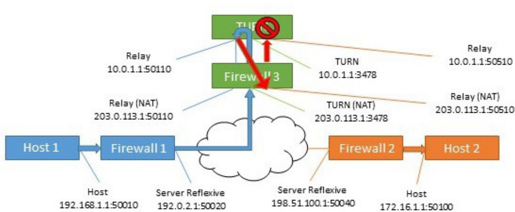
図 31 : ホスト間のメディアパス (リレー間パスを使用、NATあり)
