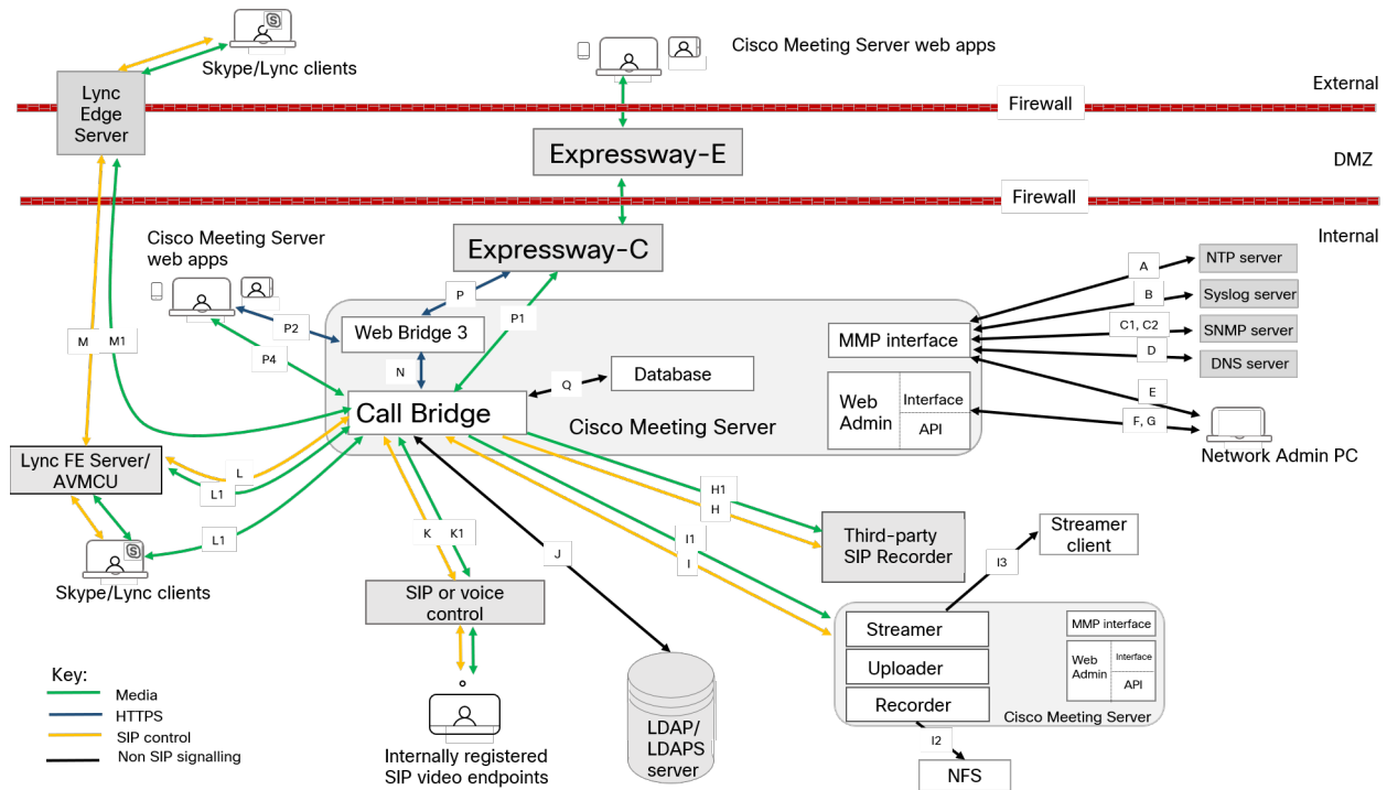
図 23 : DMZ内のExpresswayを含む統合サーバ展開で開く必要があるポート
