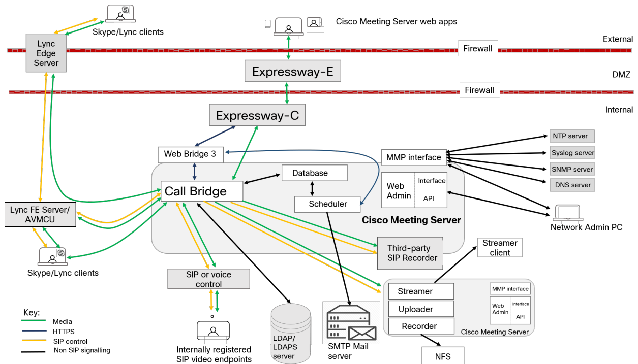
図 6 : エッジに Cisco Expressway を配置したミーティングサーバの展開例
