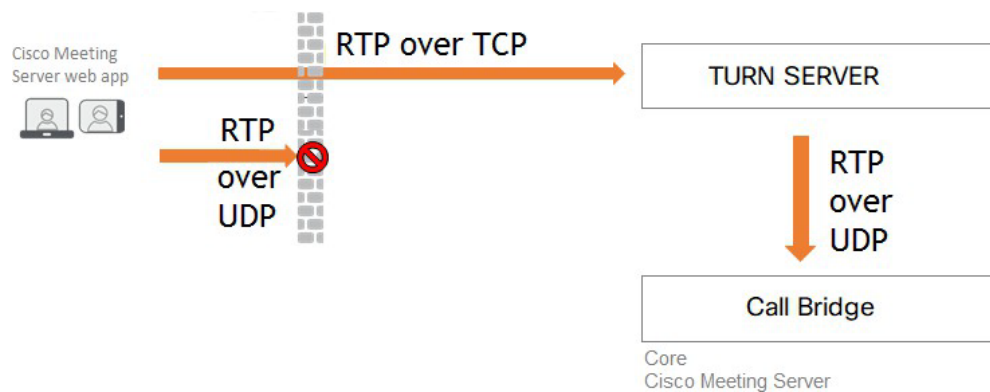
図 7：TCP および UDP をサポートする TURN サーバー
