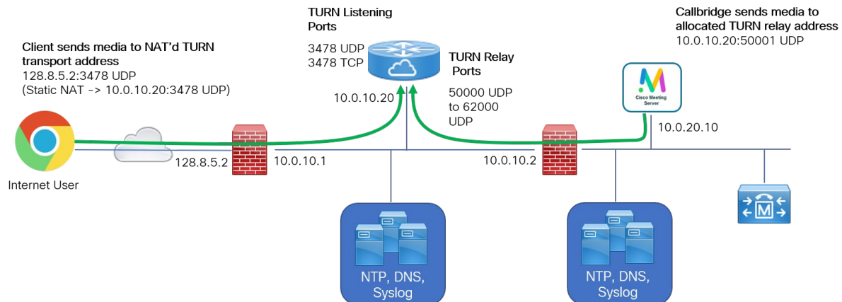
図 2 : Meeting Server Edge TURN サーバーの例
