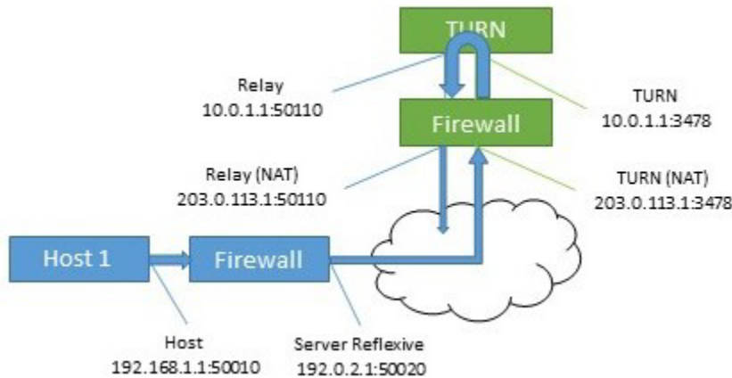
図 29 : 遠端にパケットを送信するホスト
