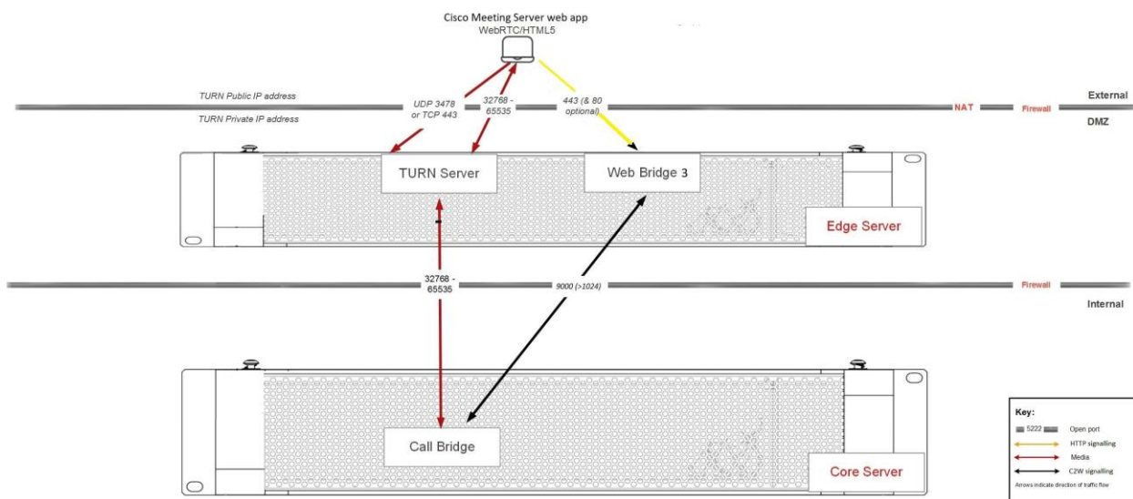
図 17: ウェブアプリのポートの使用状況
