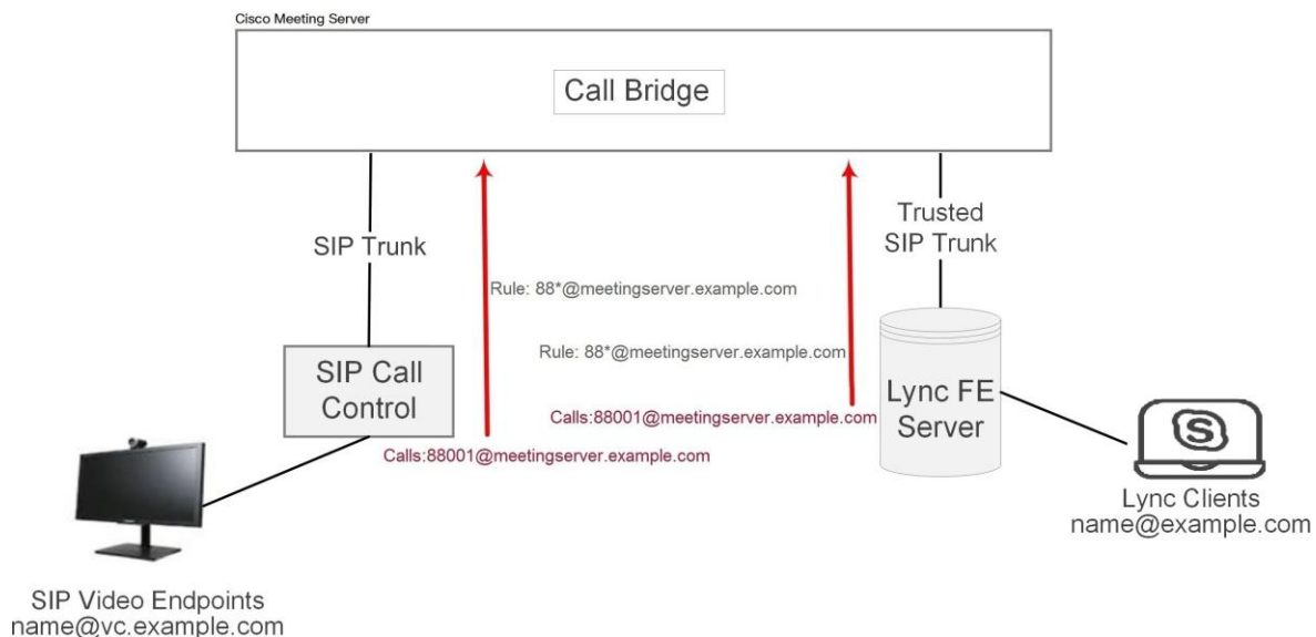
図 14： Meeting Server がホストするミーティングに参加する SIP ビデオエンドポイントと Lync クライアントの例
