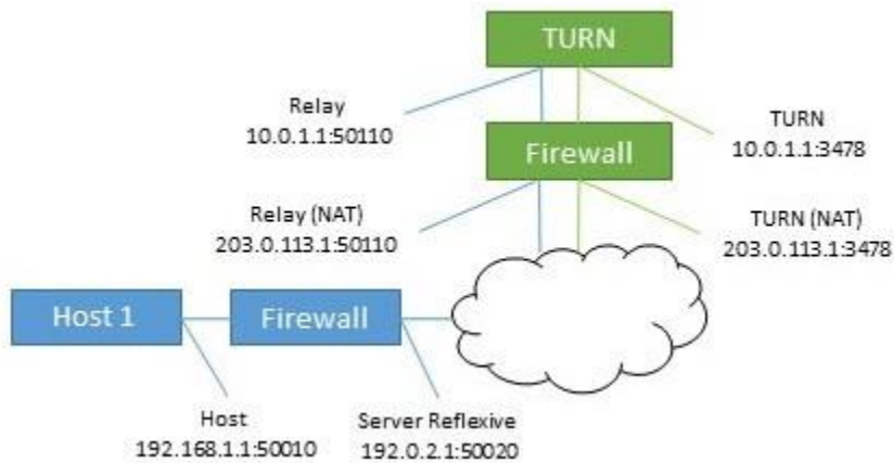
図 28: リレー候補者
