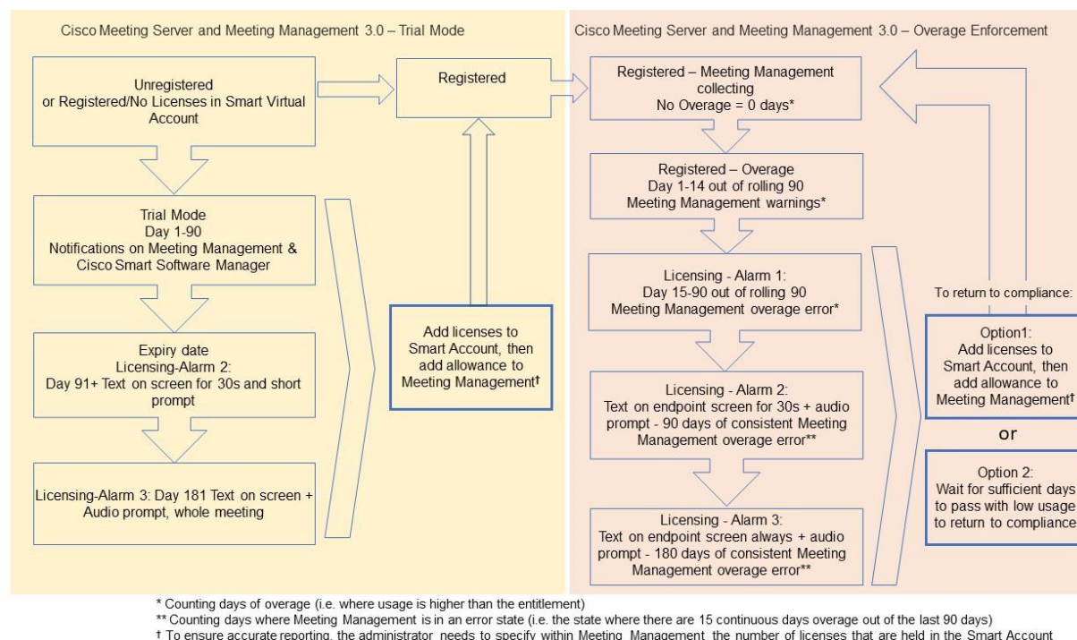
図 21 : Cisco Meeting Server および Cisco Meeting Management Smart Licensingの強制フロー
