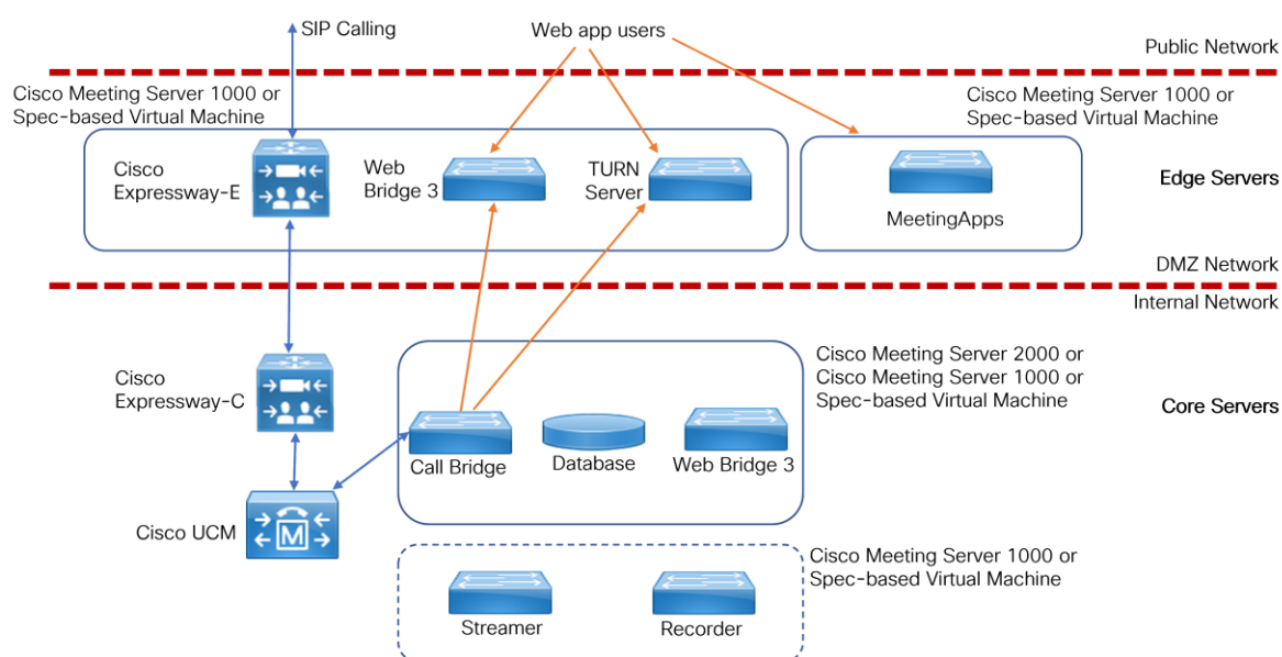
図 2 : Meeting Server Edge を使用した分割サーバ導入
