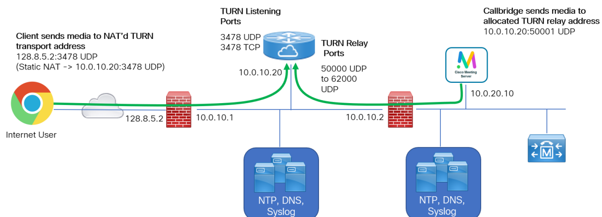
図 3 : Meeting Server Edge TURN サーバーの例
