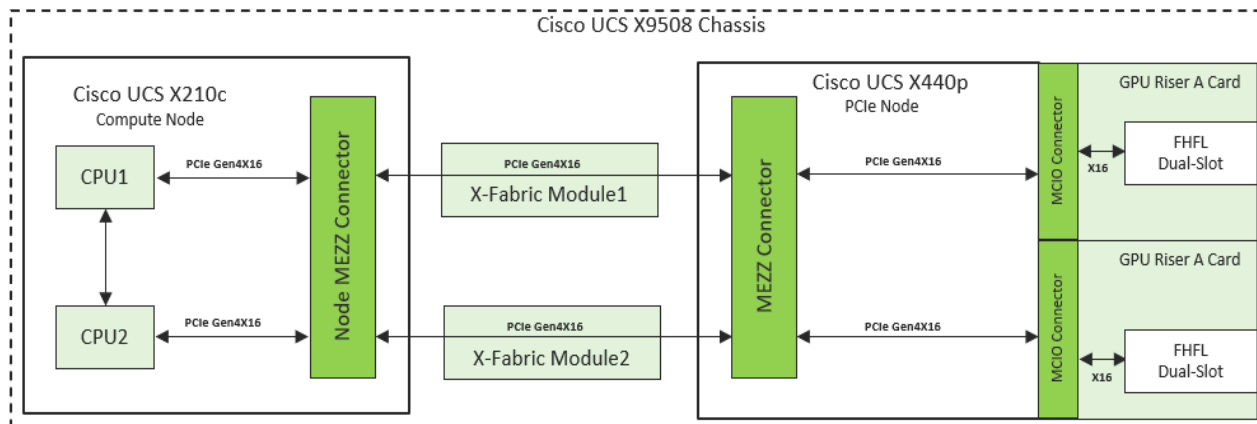
図 3 ライザー A を使用した Cisco UCSX-440P PCIe ノードの 簡略ブロック図
