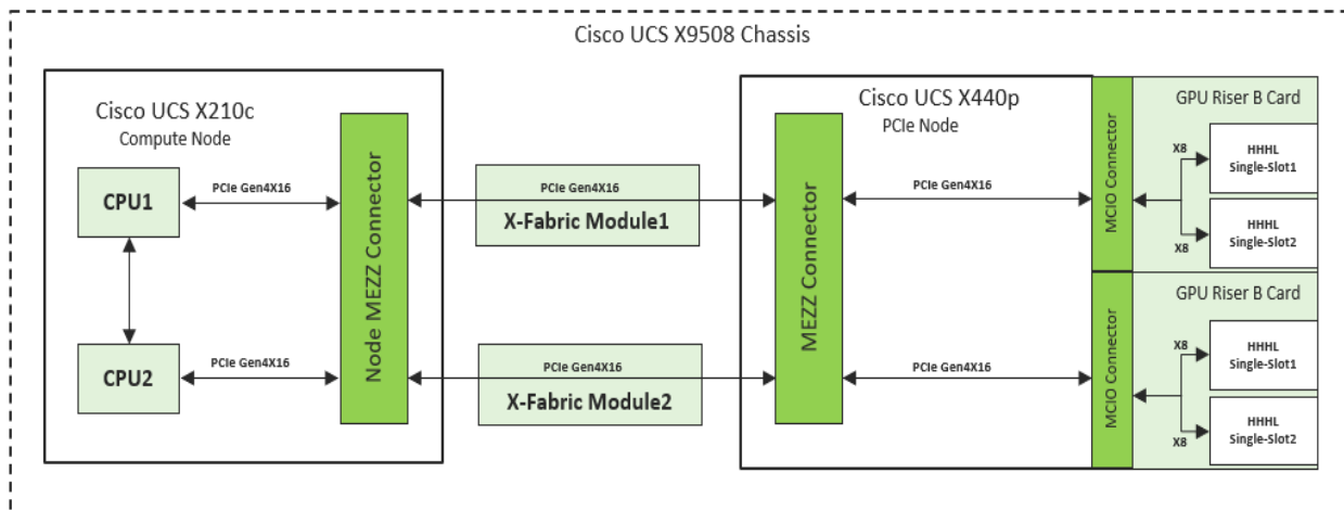
図 4 ライザー B を使用した Cisco UCS X440p PCIe ノードの簡略ブロック図
