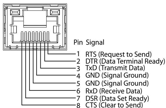
図 5 シリアル ポート (RJ-45 のメス コネクタ) のピン割り当て Serial Port (RJ-45 Female Connector)
