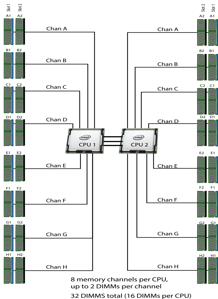
図 4 メモリ構成
