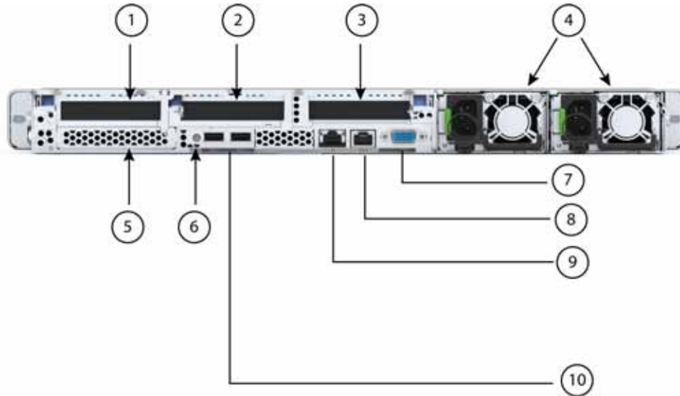
図 3 シャーシ背面図 (3つのハーフ高さ、長さ 3/4 の PCIe ライザー)
