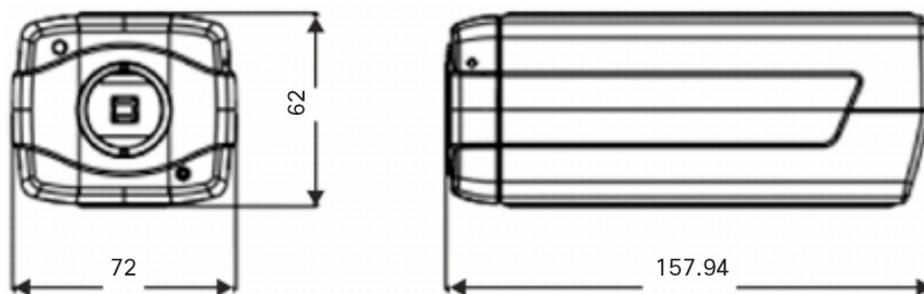
図 2. Cisco Video Surveillance 6500PD IP カメラの寸法
