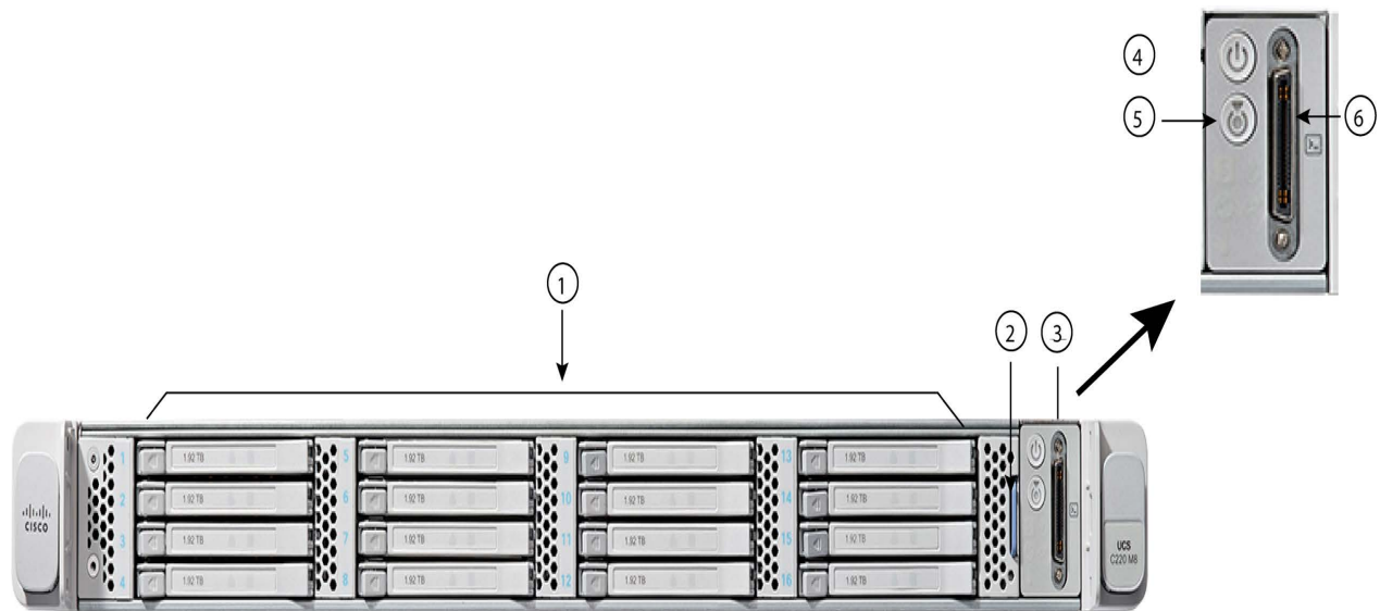
図 2 シャーシの詳細な正面図
