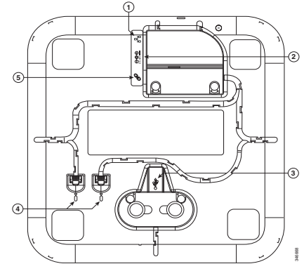
Vista inferiore dell'unità Sound Base
