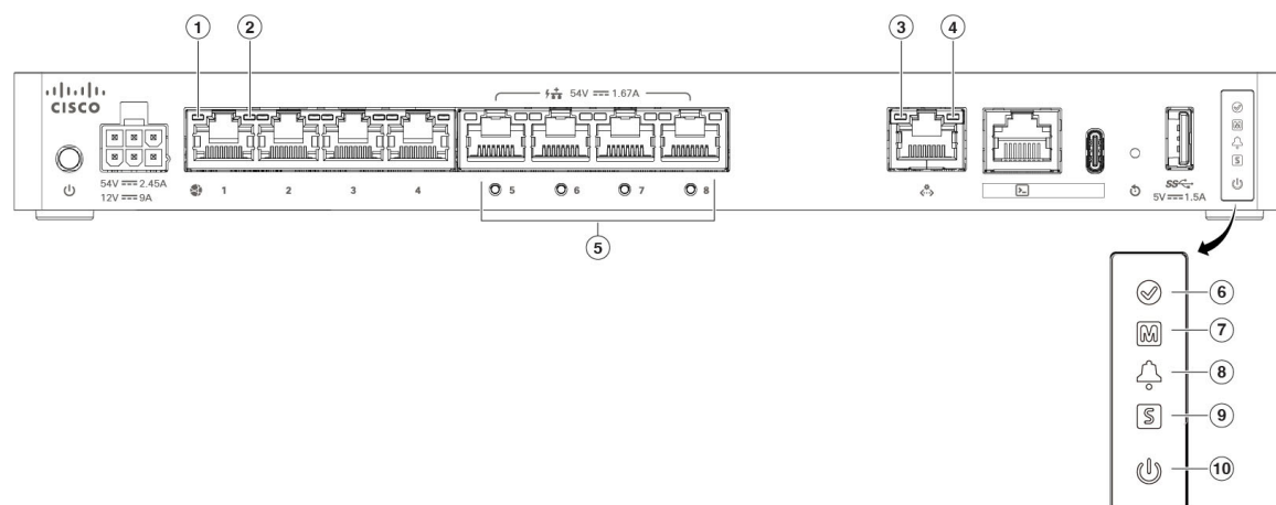
Illustration 10 : Voyants du panneau arrière du modèle Secure Firewall CSF-1210CP
