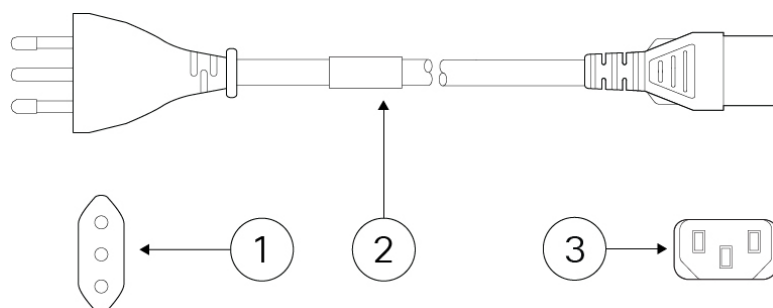
Illustration 18 : Italie (CAB-ACI)
