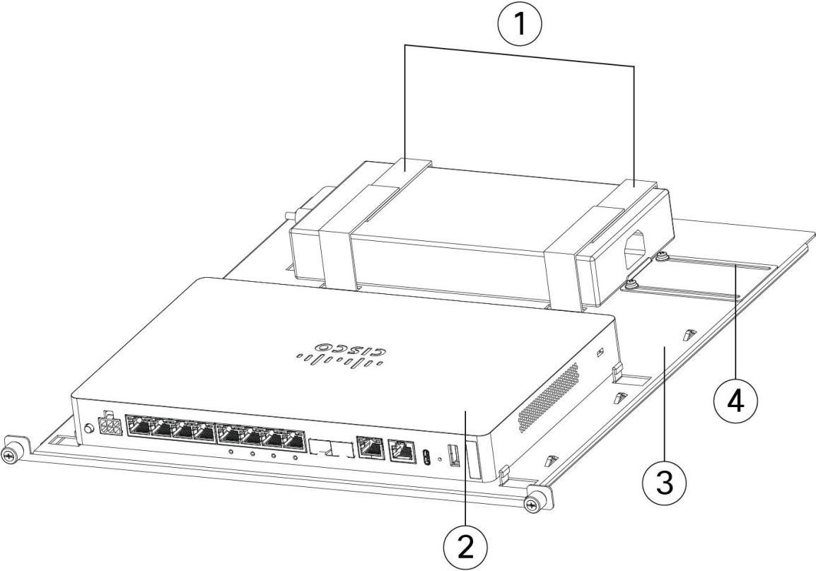
Illustration 35 : Placer le module d'alimentation sur le plateau coulissant et serrer les bandes Velcro
