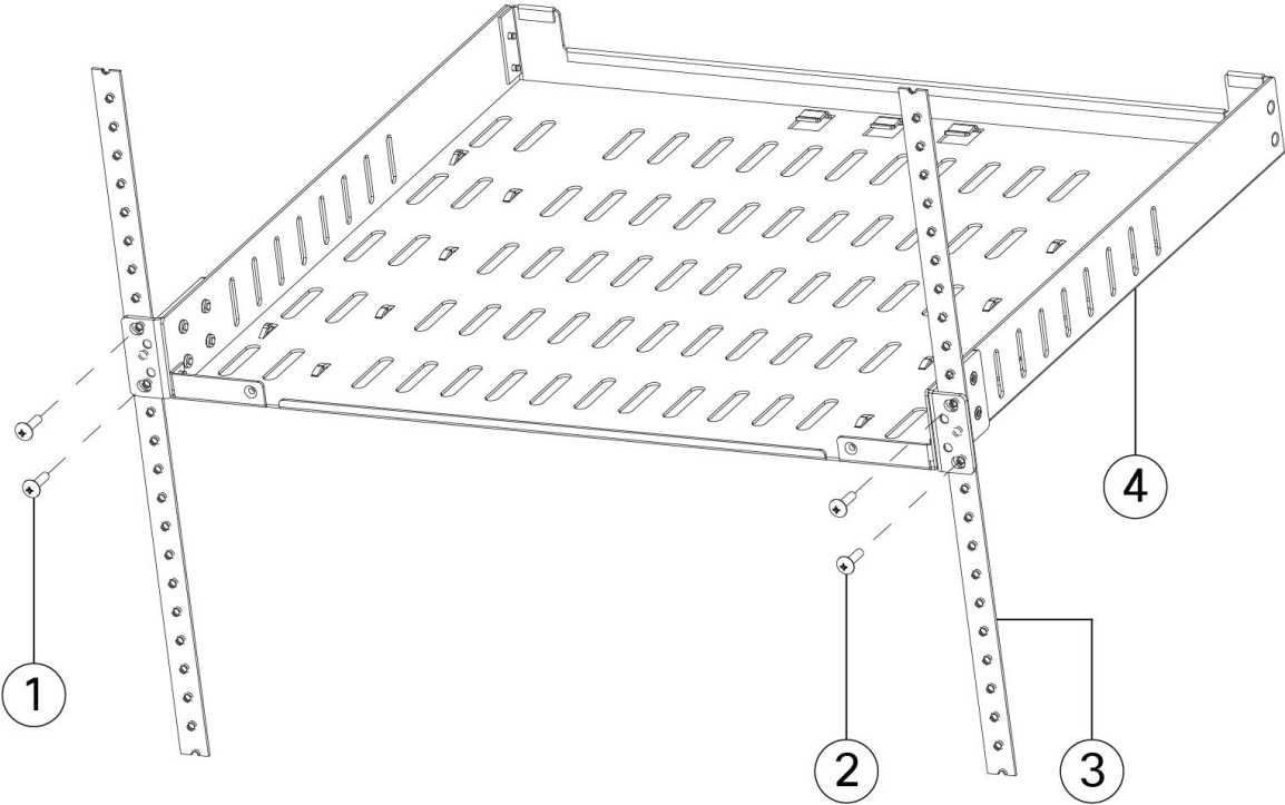
Illustration 33 : Installer la tablette de montage dans le rack
