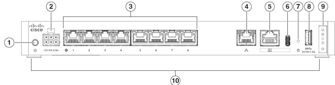
Illustration 6 : Panneau arrière du modèle Secure Firewall CSF-1210CE
