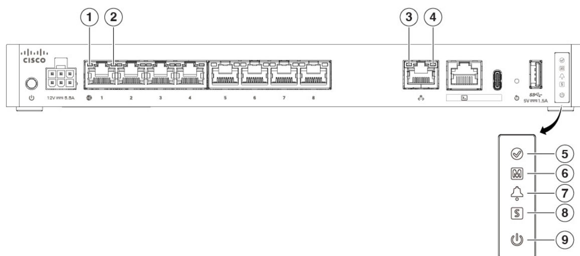
Illustration 9 : Voyants du panneau arrière du modèle Secure Firewall CSF-1210CE
