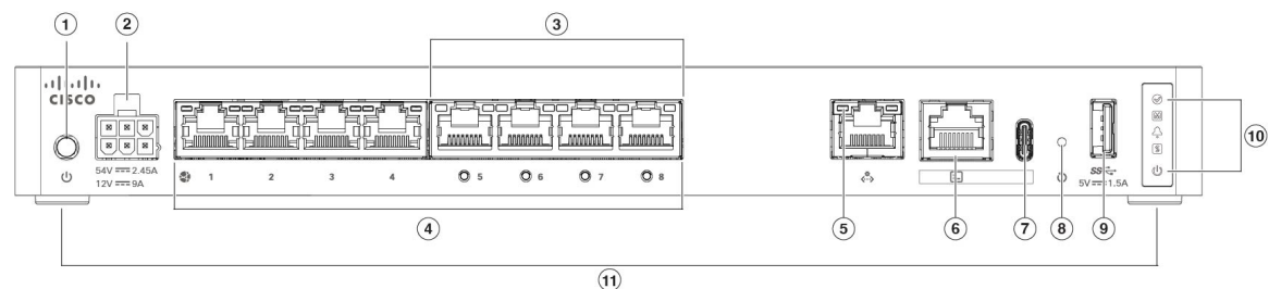
Illustration 7 : Panneau arrière du modèle Secure Firewall CSF-1210CP
