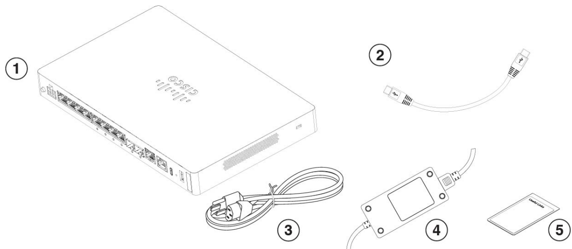
Illustration 2 : Contenu du coffret des modèles Secure Firewall CSF-1210CE, CSF-1210CP et CSF-1220CX
