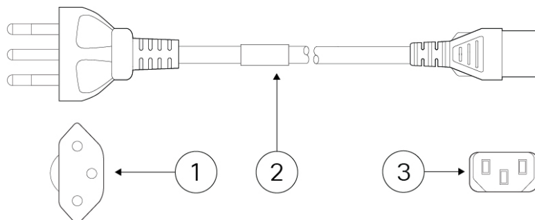
Illustration 25 : Suisse (CAB-ACS)
