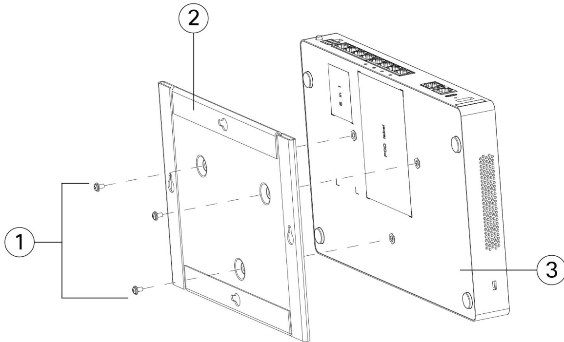
Illustration 31 : Fixation du support de montage mural au châssis
