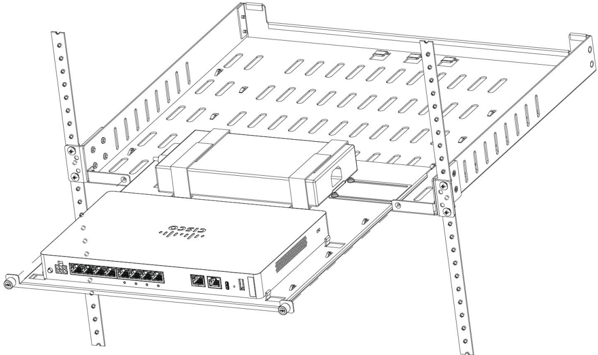
Illustration 36 : Faire glisser le plateau coulissant dans la tablette de montage en rack
