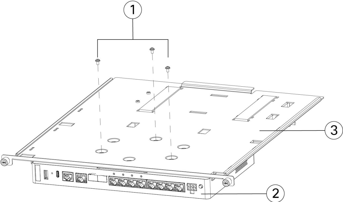
Illustration 34 : Installer le plateau coulissant sur le châssis
