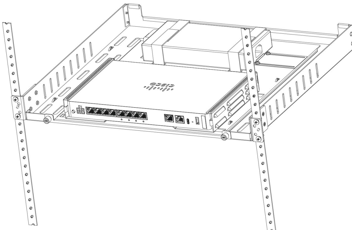
Illustration 37 : Plateau coulissant installé sur la tablette de montage en rack
