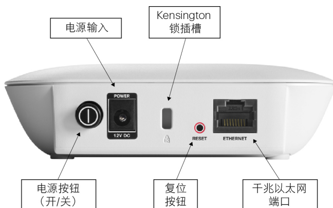
图 3. 支持单点设置的 Cisco WAP321 Wireless-N 可选频段接入点的后面板
