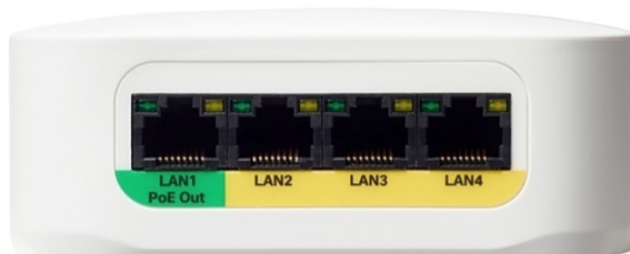
Abbildung 4. Seitenteil des WAP361 Wireless-AC/N Dual Radio Wall Plate Access Point
