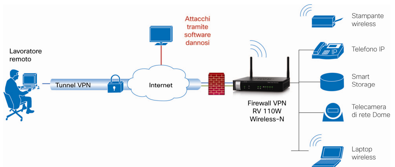
Figura 3. Configurazione tipica del Firewall VPN Cisco RV110W Wireless-N
