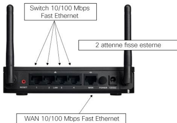
Figura 3. Configurazione tipica del Firewall VPN Cisco RV110W Wireless-N
