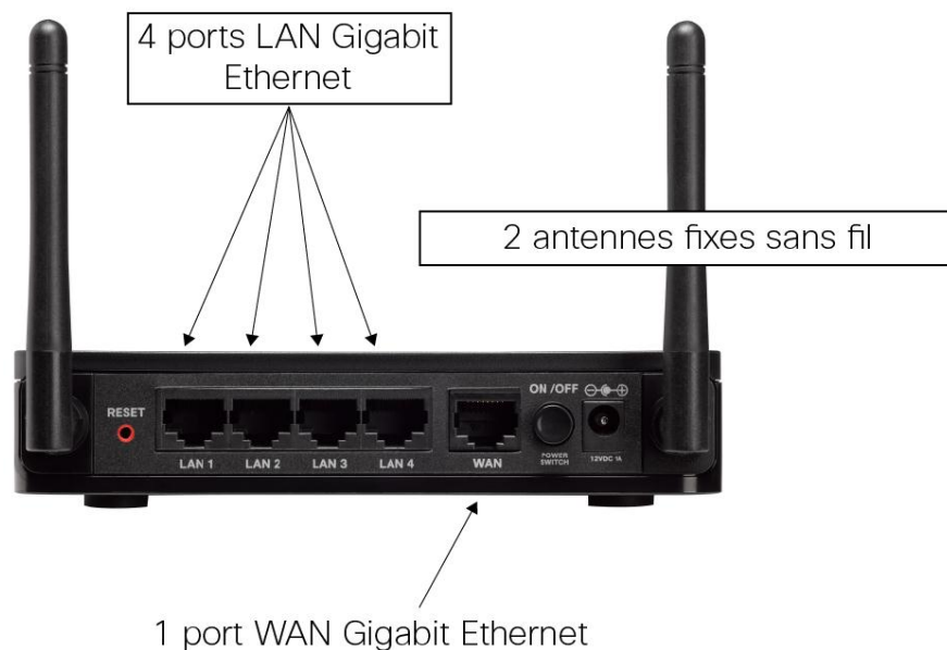
Donnée 2. Routeur VPN multifonction Cisco RV180W (vue arrière)
