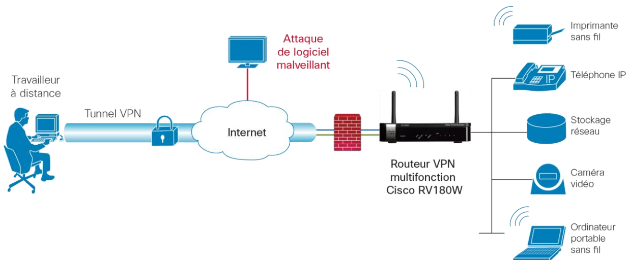
Donnée 3. Configuration usuelle pour routeur VPN multifonction Cisco RV180W
