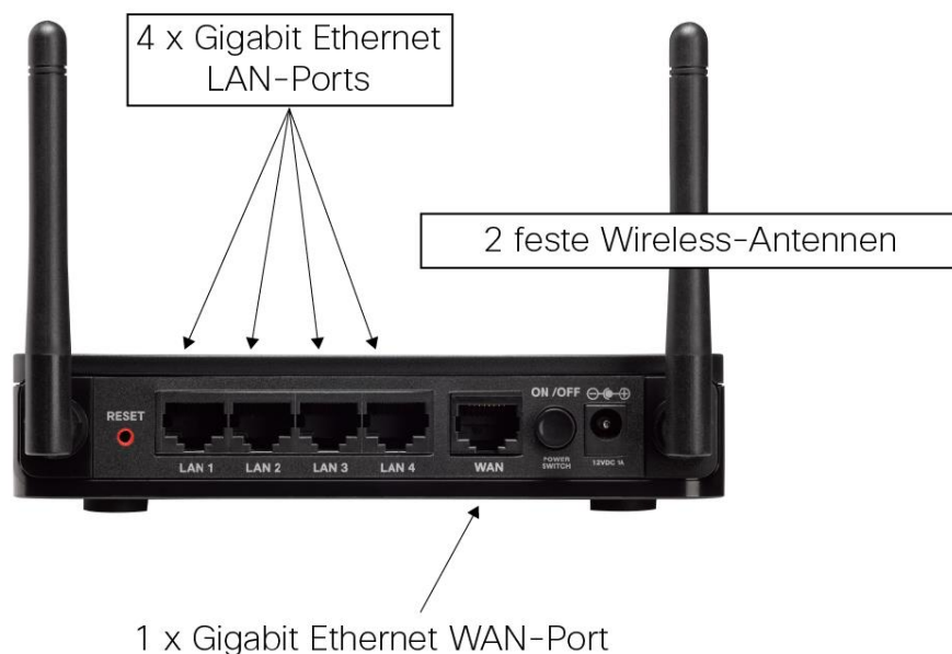
Abbildung 2. Cisco RV180W Multifunktions-VPN-Router (Rückseite)
