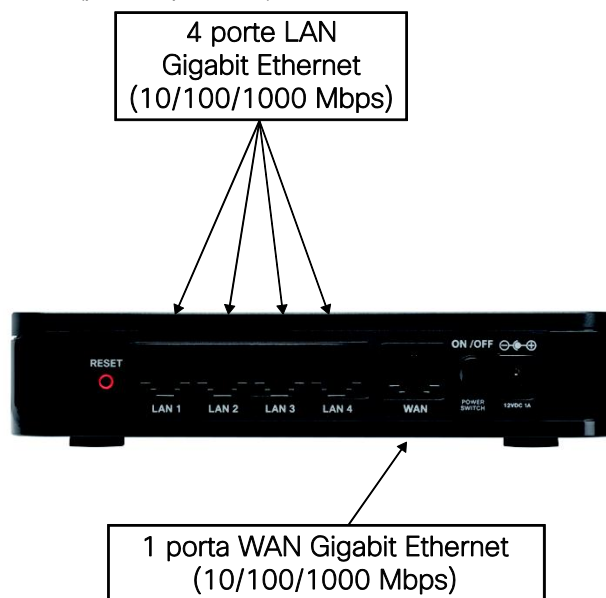
Figura 2. Router VPN Cisco RV180 (pannello posteriore)
