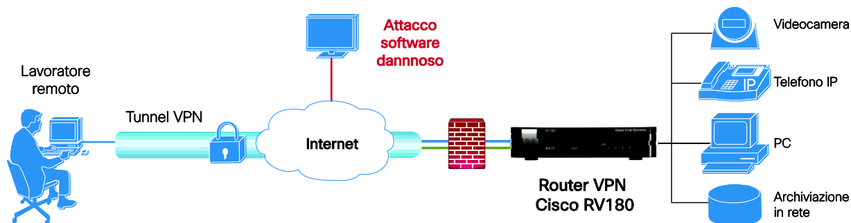
Figura 3. Configurazione tipica del router VPN Cisco RV180
