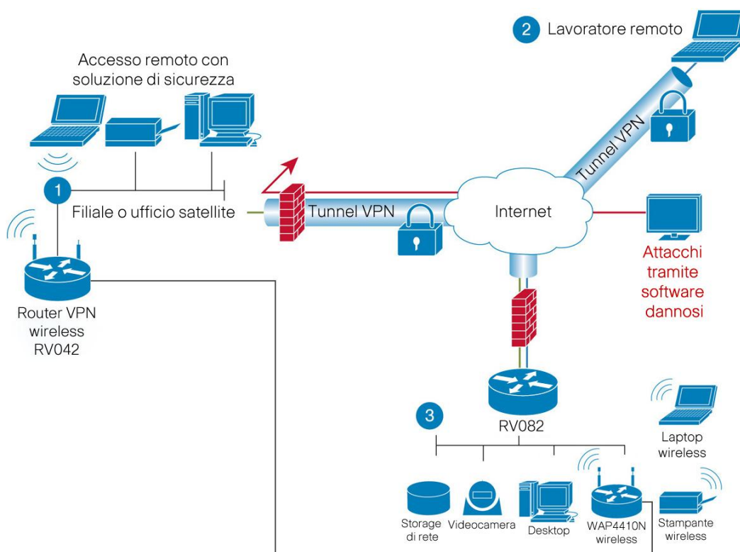
Figura 3. Configurazione tipica
