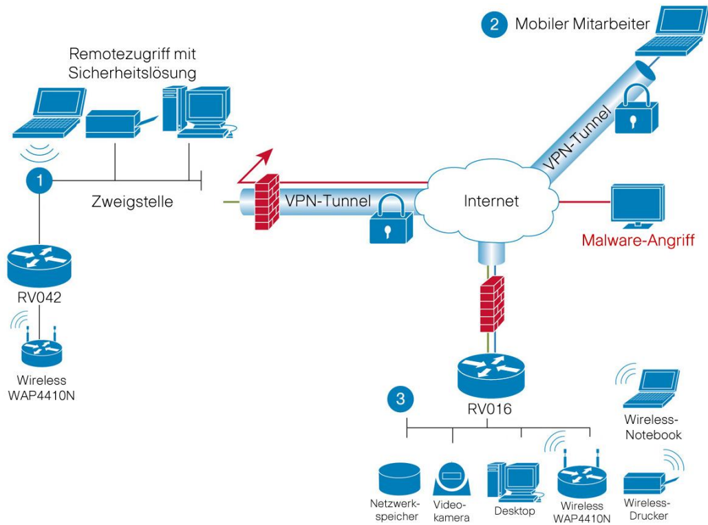
Abbildung 3. Typische Konfiguration
