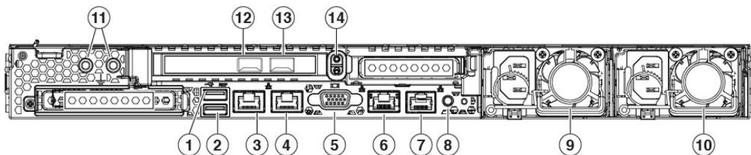
4600 و 2600 و FMC 1600 ةيفلخل ةحول 3. لكش
