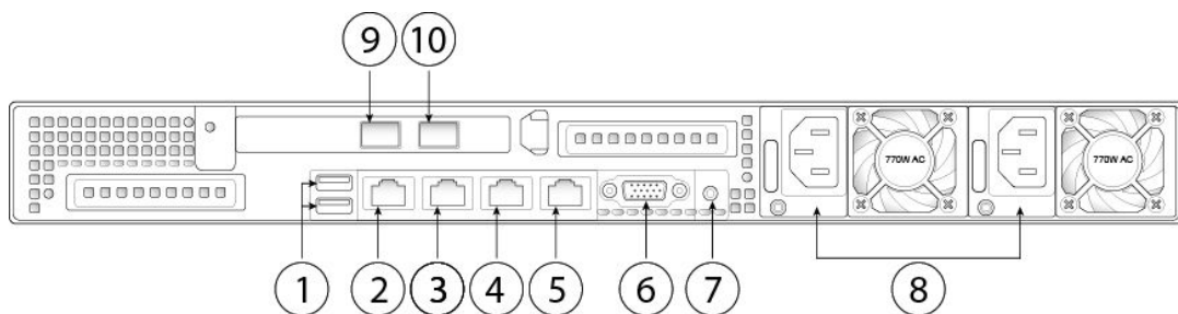
4500 و FMC 2500 ةيفلخلال ةحول 2. لكش
