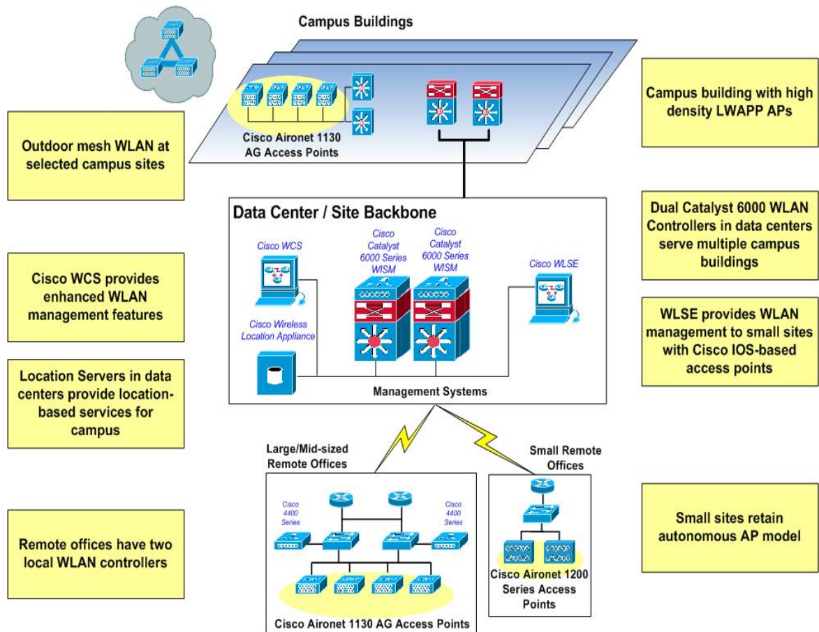
Figure 1. シスコ本社キャンパスから小規模営業オフィスまでに至るシスコ WLAN アップグレードの全体的なアーキテクチャ
