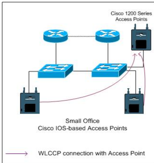
Figure 4. 自律的オペレーションと管理による分散型の WLAN デザインがとられる小規模オフィス。
