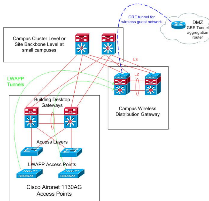
Figure 2. キャンパスサイトでのシスコの次世代 WLAN アーキテクチャのデザイン
