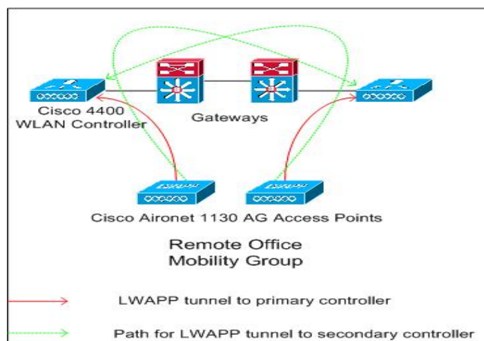
Figure 3. 中央管理型のアーキテクチャをベースとした大規模および中規模営業オフィスの WLAN デザイン
