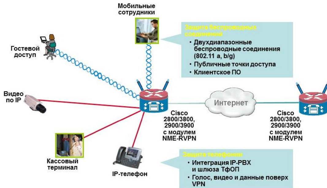
Рисунок 3. Защита беспроводных и мультисервисных сетей
