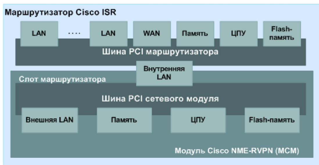
Рисунок 4. Архитектура модуля NME-RVPN (MCM) и маршрутизатора Cisco ISR
