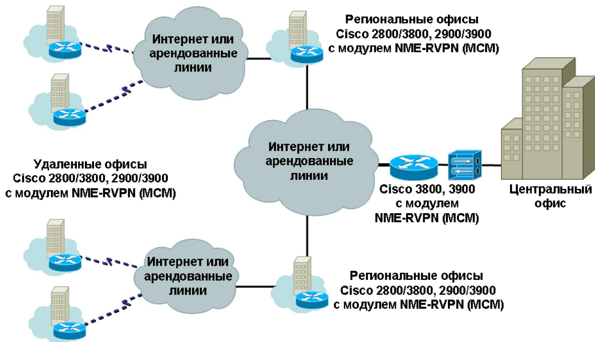
Рисунок 2. Использование VPN туннелей для создания защищенной корпоративной сети
