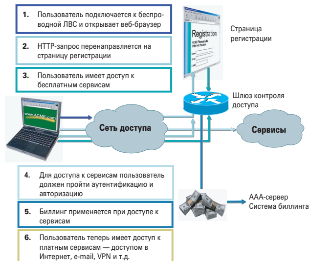
Рис. 6 Процедура доступа пользователей к сервисам
