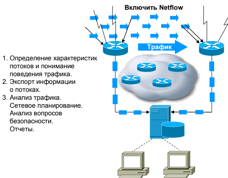
Рисунок 4. Принципы работы Cisco NetFlow
