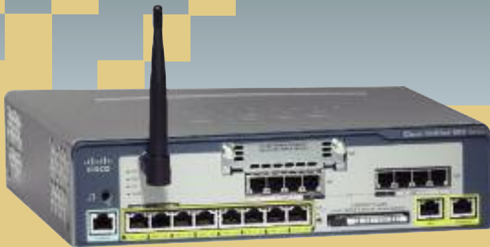
Базовый модуль с поддержкой сетей Wi-Fi (модель с 4 аналоговыми городскими линиями, 4 внутренними портами для аналоговых телефонов и модулем расширения на 4 дополнительных аналоговых порта)
