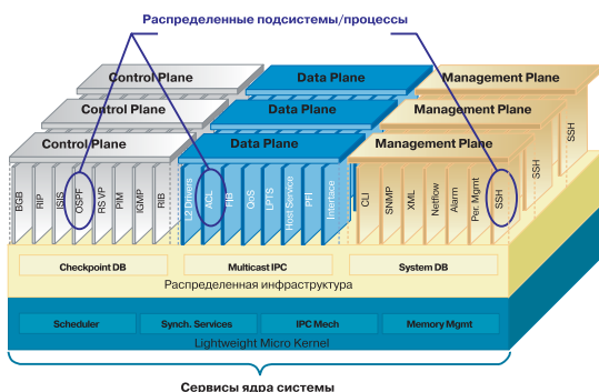
Рисунок 4. Архитектура Cisco IOS XR
