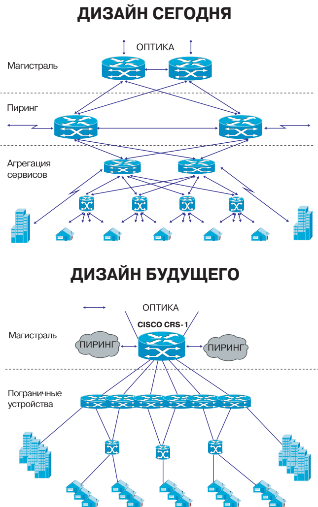
Рисунок 3. Упрощение архитектуры с помощью Cisco CRS-1
