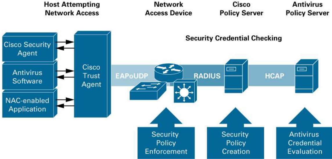
그림 1 CTA 아키텍처 개요
