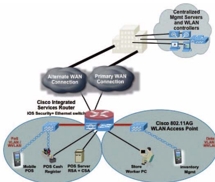
小規模の小売店舗：検証済みのネットワーク設計
