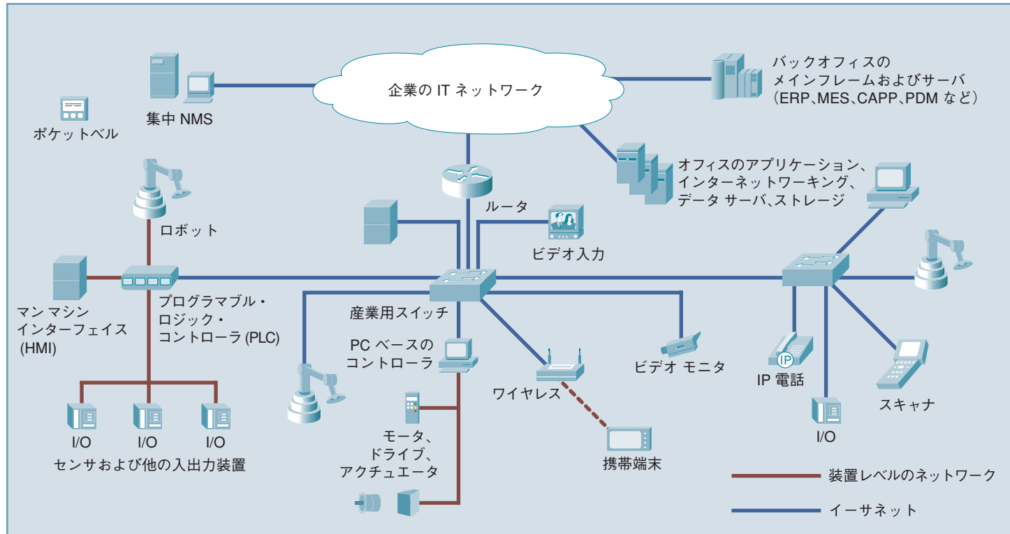
図1 ネットワーク ダイアグラム
