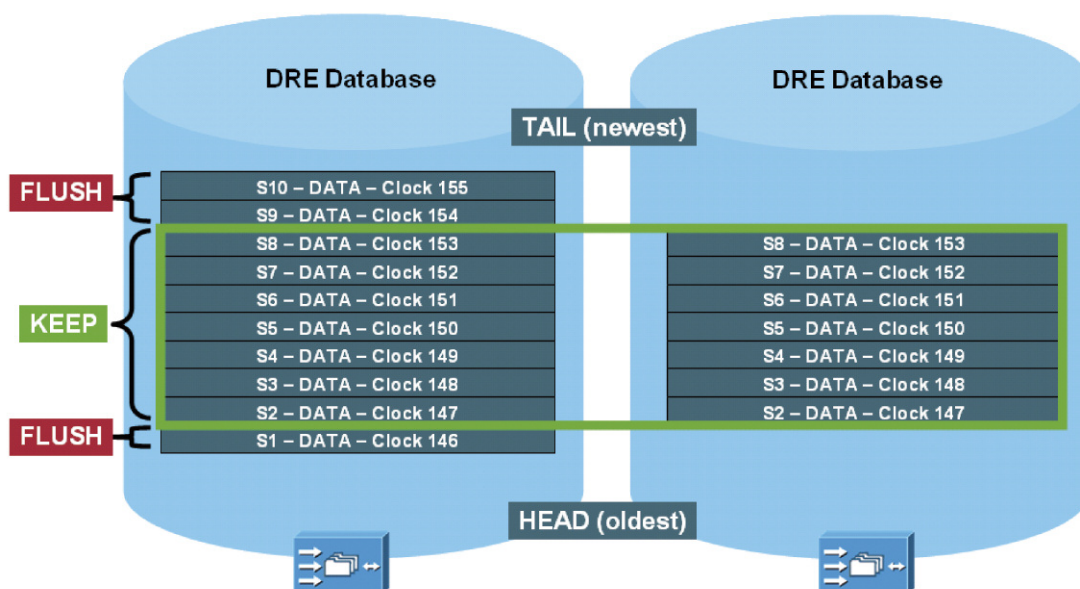
Figure 9 : Synchronisation des contextes DRE
