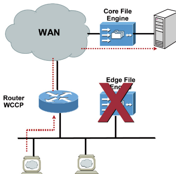
Figure 21 : Bypass WCCP en cas de défaillance des WAE
