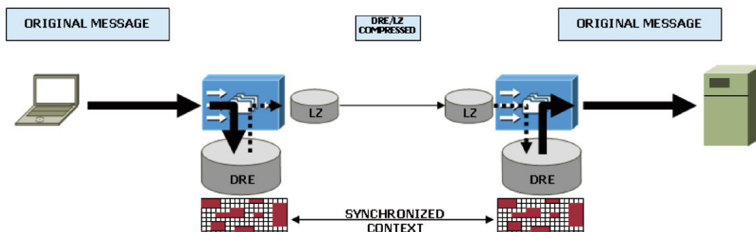
Figure 6 : Représentation globale des mécanismes de compression
