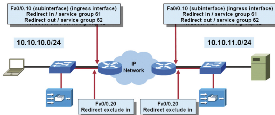
Figure 19 : Points de redirection sur les routeurs pour le trafic entrant et sortant
