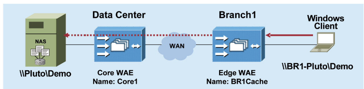
Figure 25 : Connexion d'un client CIFS en mode proxy
