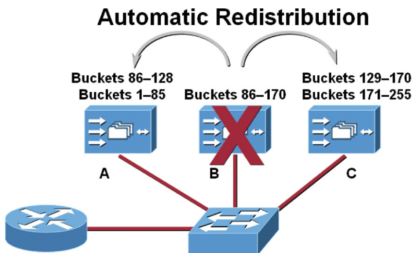
Figure 15 : Algorithme de partage de charge WCCP
