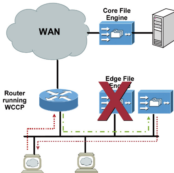
Figure 22 : Redistribution de la charge en cas de défaillance d'un WAE
