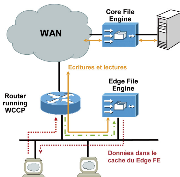
Figure 18 : Propagation de la requêtes en central en cas de "cache miss"
