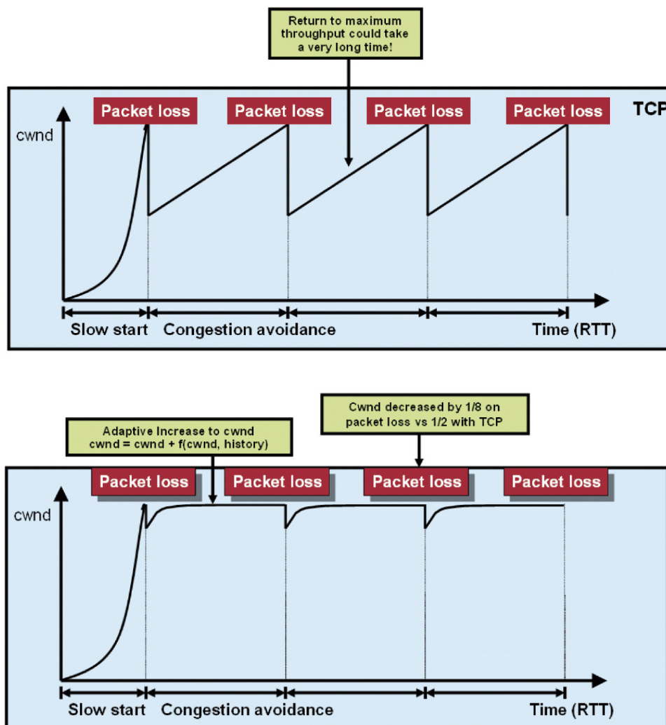
Figure 5 : Action de «l'adaptive increase windows size»
