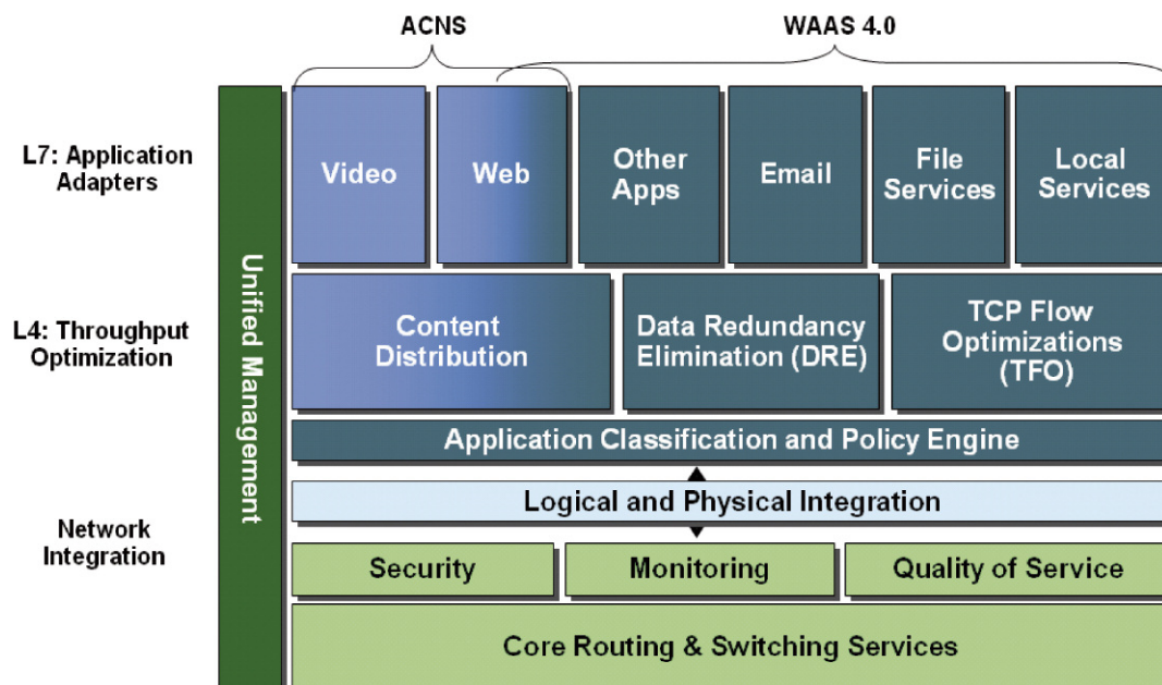
Figure 1 : Services WAAS et ACNS
