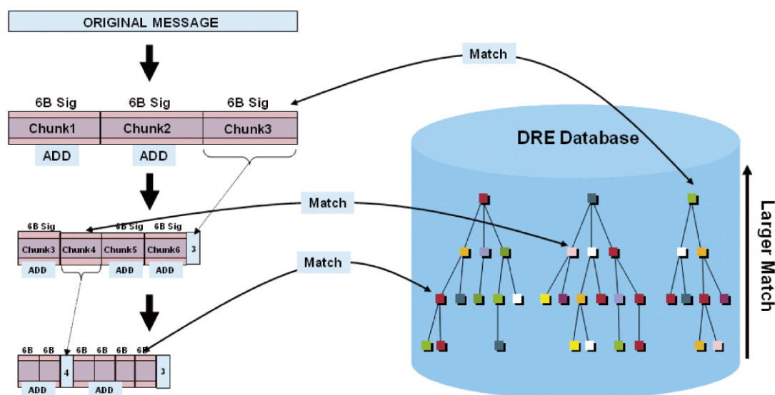
Figure 7 : Base de données DRE
