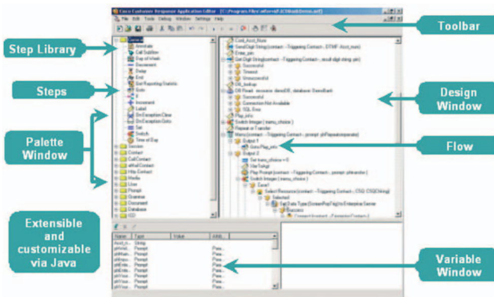
Abbildung 3: Umgebung für Service-Erstellung und Scripting
