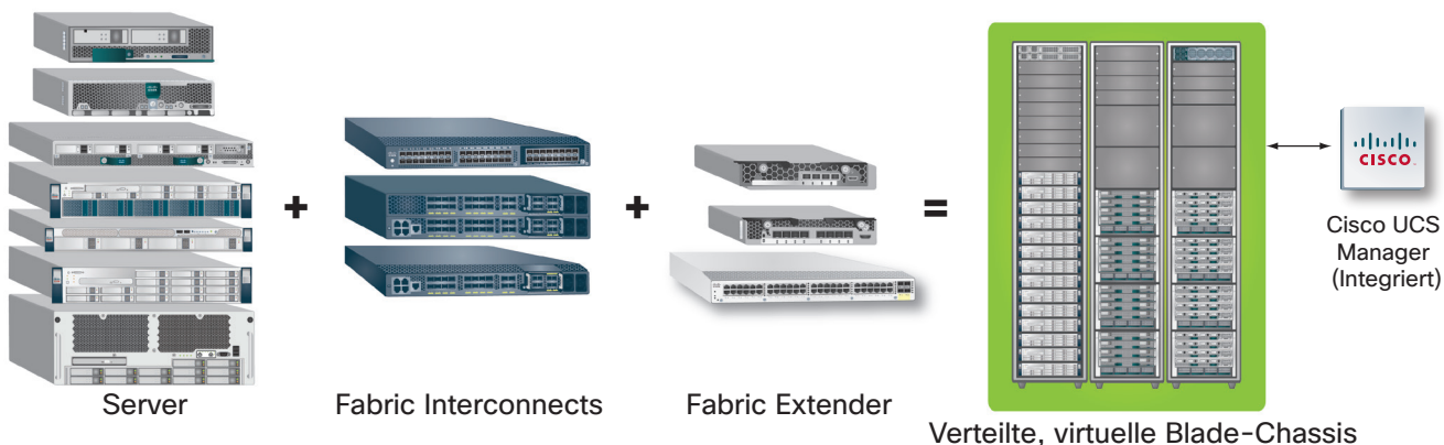
Abbildung 2. Das Cisco UCS kombiniert Blade- und Rack-Server sowie Netzwerk- und Speicherressourcen in einem verteilten, virtuellen Blade-Chassis mit einem zentralen, redundanten Anbindungs- und Managementpunkt
