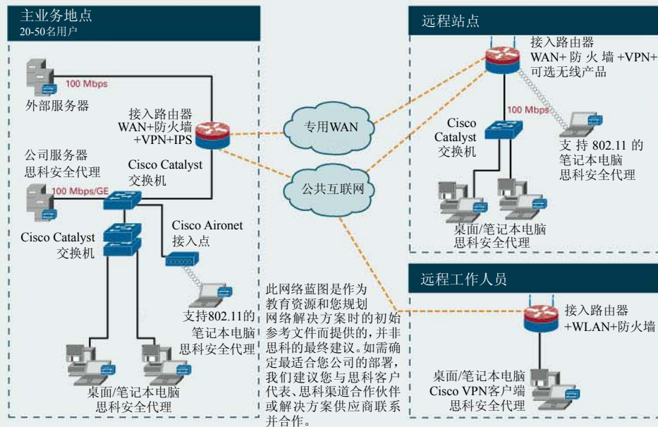
图 1: 中小型企业网络蓝图（每站点 20 到 50 个用户端口）
