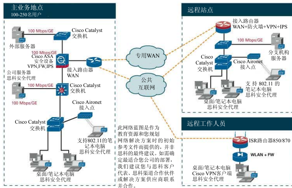
图 3: 中小型企业网络蓝图(每站点 100 到 250 个用户端口)
