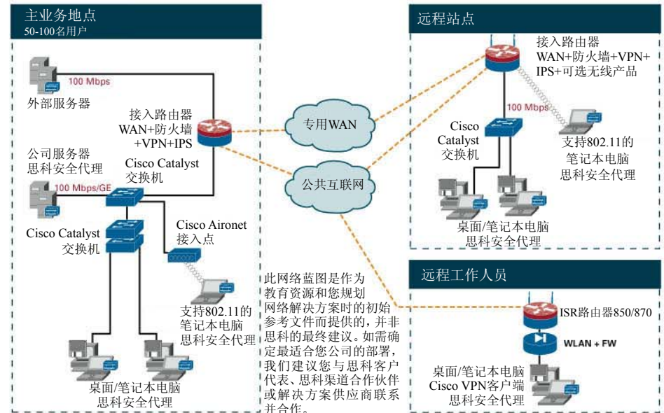
图 2: 中小型企业网络蓝图（每站点 50 到 100 个用户端口）
