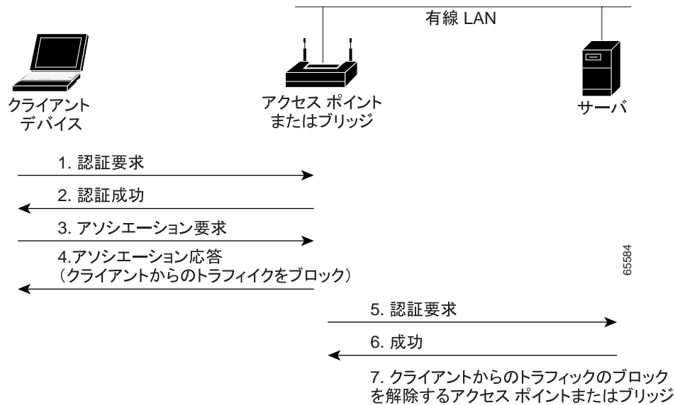
図 11-4 MAC ベースの認証のシーケンス
