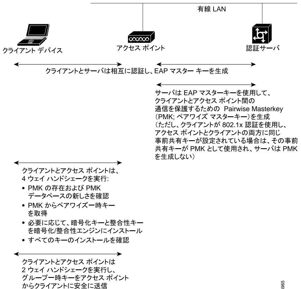
図 11-6 WPA キー管理プロセス
