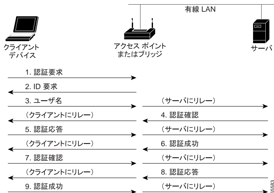
図 11-3 EAP 認証のシーケンス
