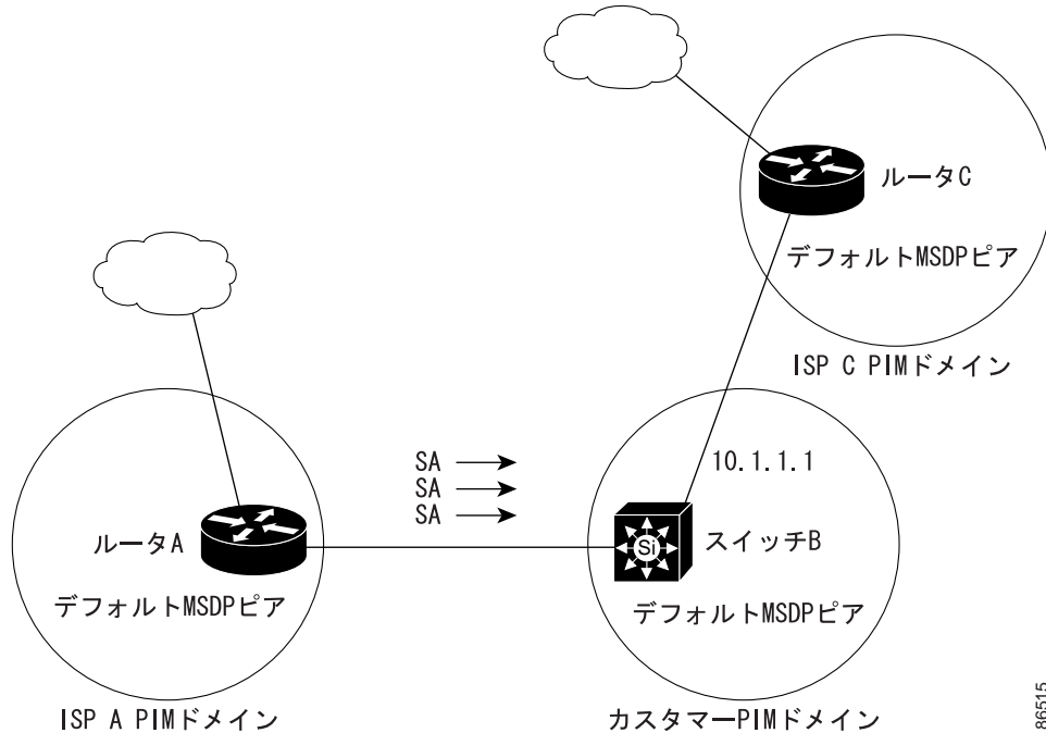
図 34-2 デフォルトの MSDP ピア ネットワーク
