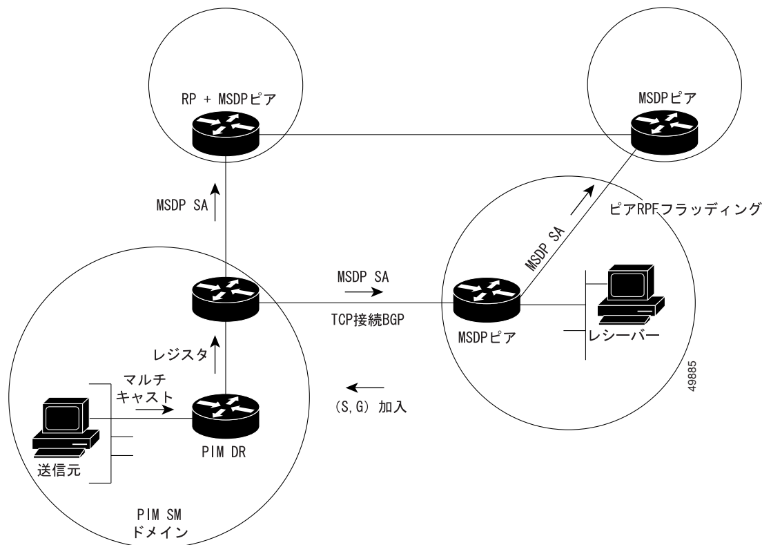
図 34-1 RP ピア間で動作する MSDP
