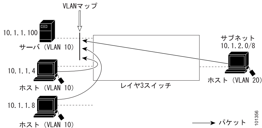
図 28-5 別の VLAN にあるサーバへのアクセス拒否
