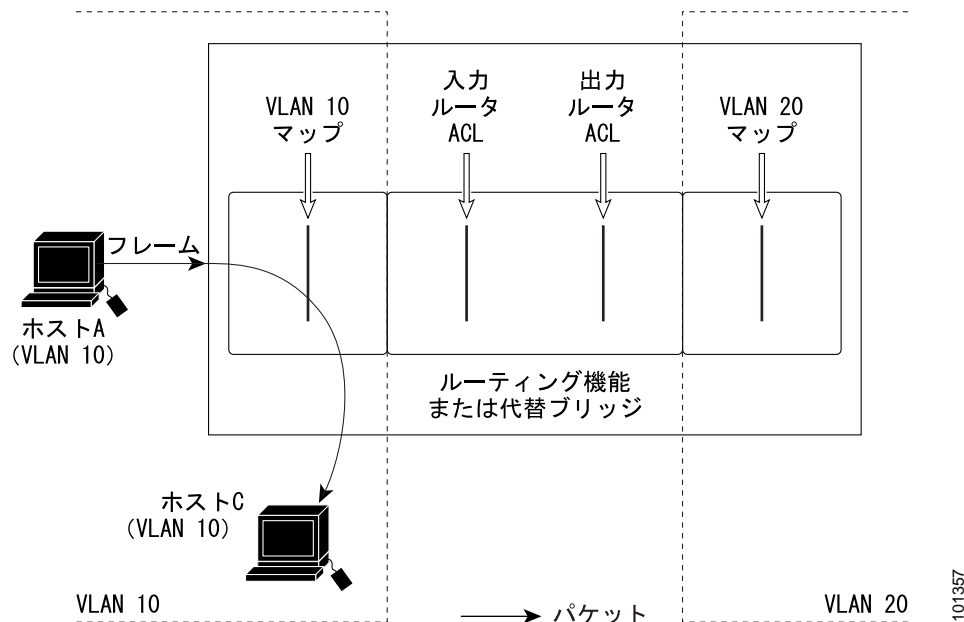
図 28-6 スイッチド パケットへの ACL の適用
