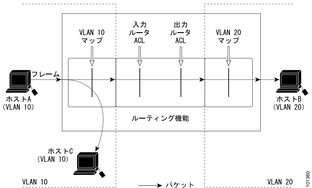
図 28-9 マルチキャスト パケットへの ACL の適用
