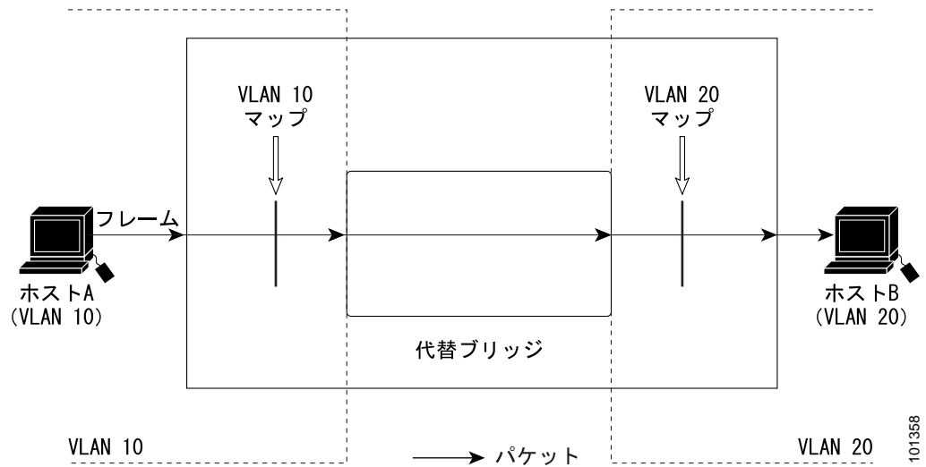
図 28-7 ブリッジド パケットへの ACL の適用
