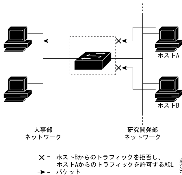
図 28-1 ACL によるネットワーク トラフィックの制御
