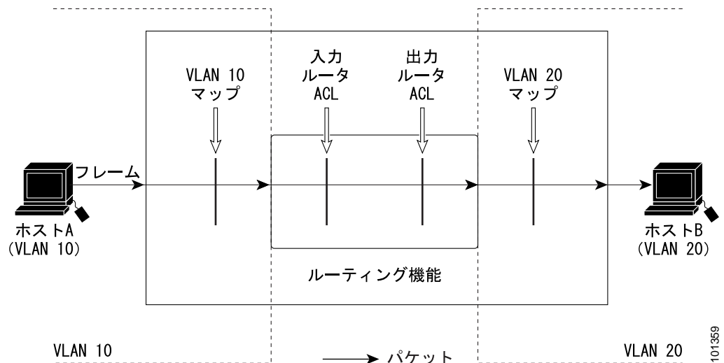
図 28-8 ルーテッド パケットへの ACL の適用
