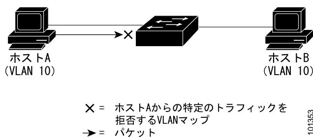
図 28-2 VLAN マップによるトラフィックの制御
