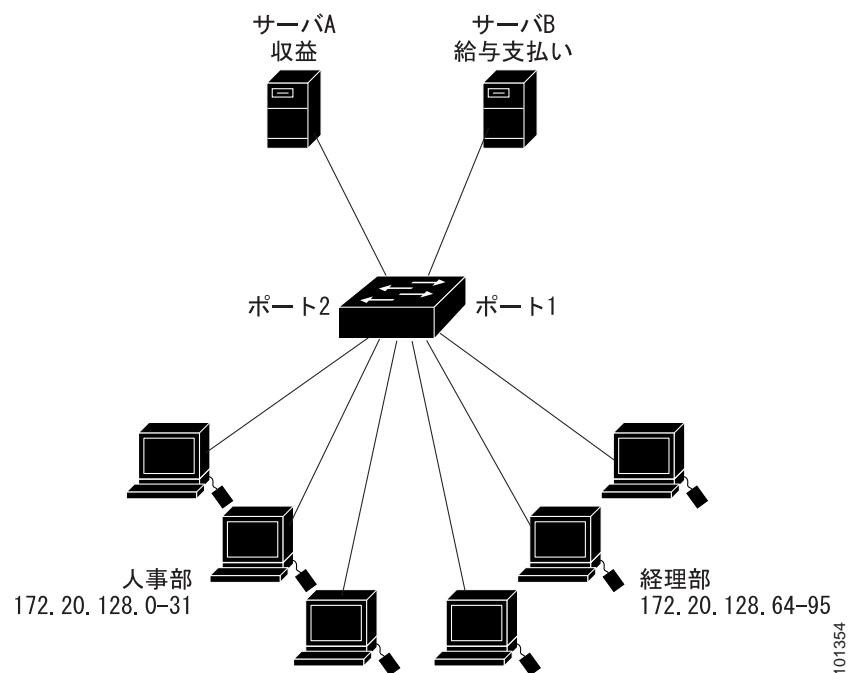
図 28-3 ルータ ACL によるトラフィックの制御
