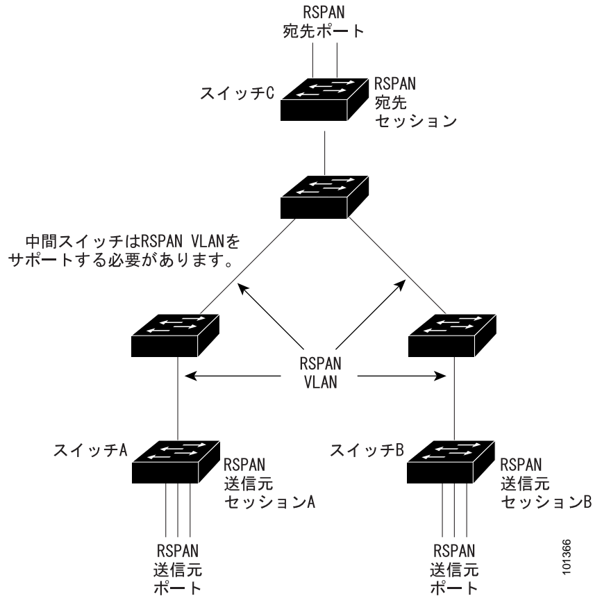
図 24-3 RSPAN の設定例
