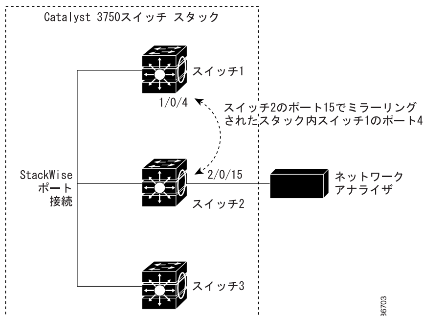
図 24-2 スイッチ スタックでのローカル SPAN の設定例
