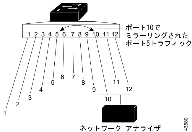
図 24-1 単一スイッチでのローカル SPAN の設定例
