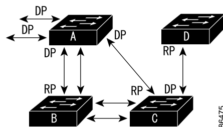
図 16-3 スパニングツリー トポロジ
