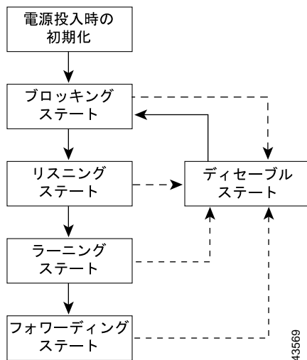
図 16-2 スパニングツリー インターフェイスのステート
