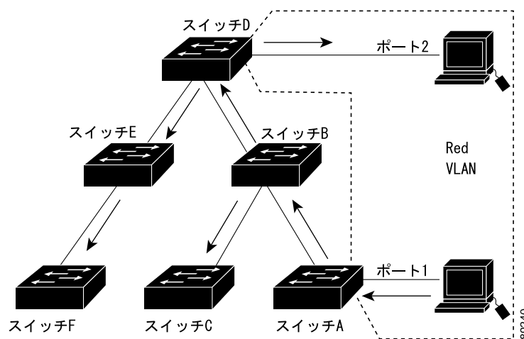
図 14-1 VTP プルーニングなしでのフラッディング トラフィック
