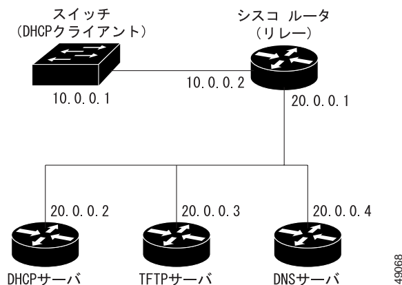
図 4-2 リレー デバイスを使用した自動設定
