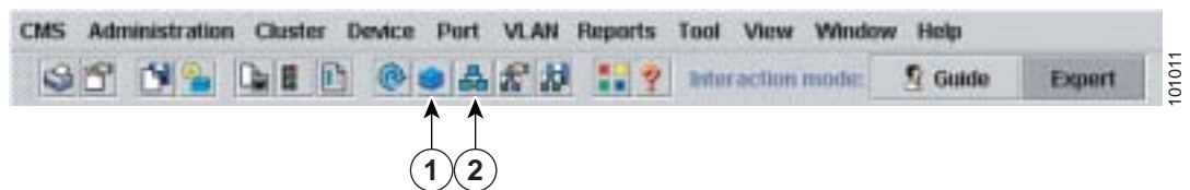
図 3-6 ツールバー
