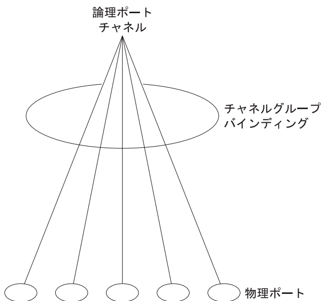
図 33-2 物理ポート、論理ポートチャンネル、およびチャンネルグループの関係
