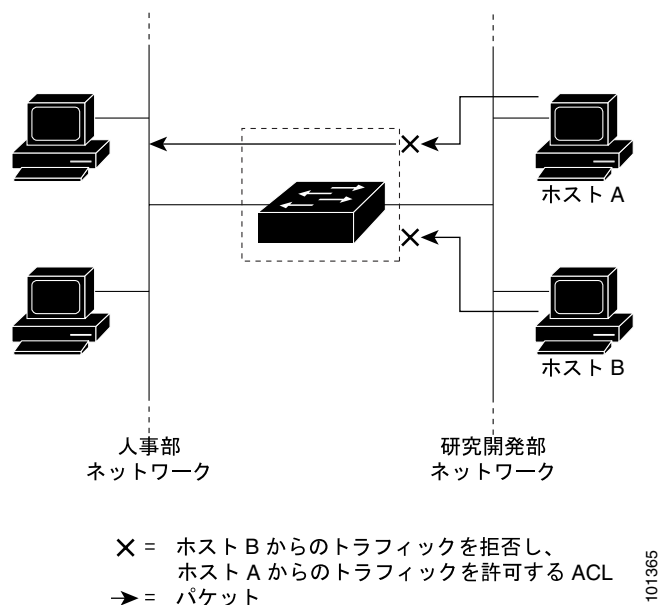
図 31-1 ACL を使用したネットワーク トラフィックの制御
