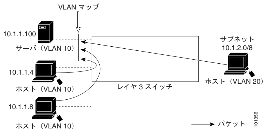
図 31-5 他の VLAN 上のサーバへのアクセス拒否
