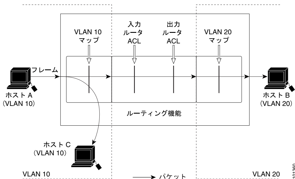
図 31-9 マルチキャスト パケットへの ACL の適用
