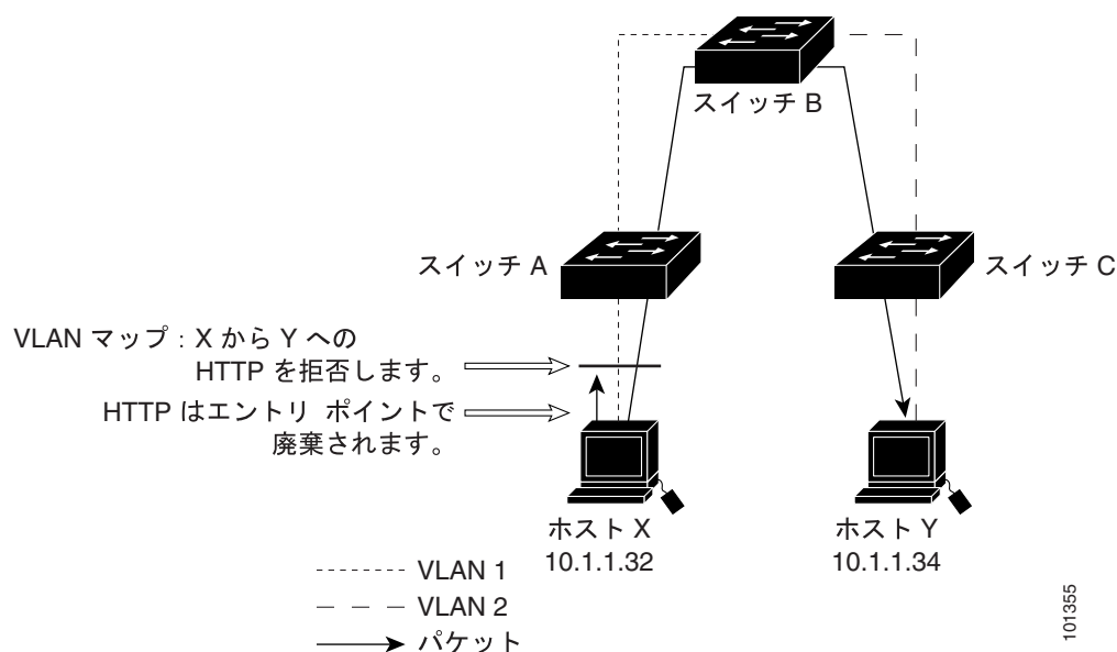
図 31-4 ワイヤリング クローゼットの設定
