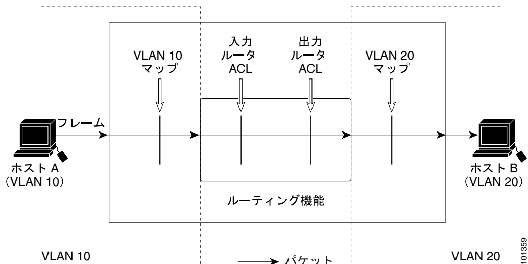
図 31-8 ルーテッド パケットへの ACL の適用
