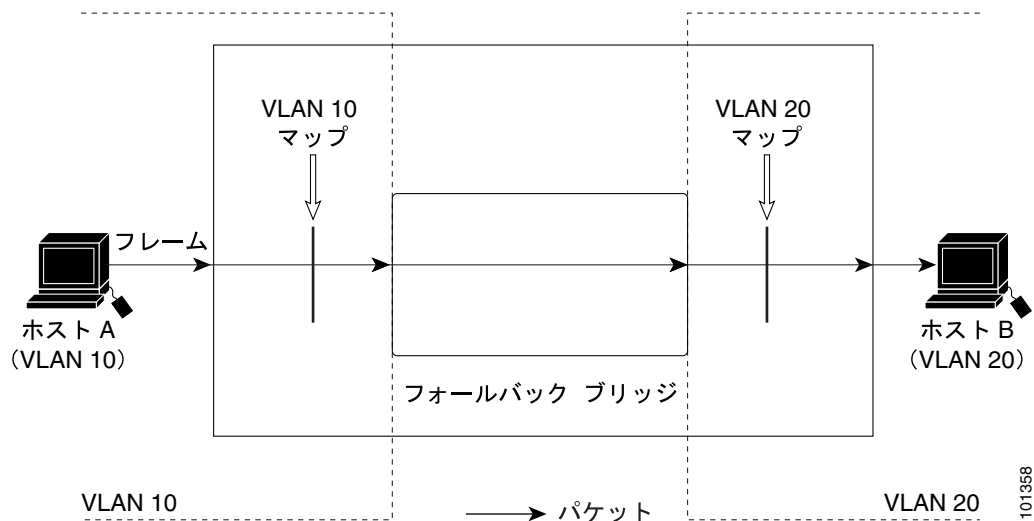
図 31-7 ブリッジド パケットへの ACL の適用
