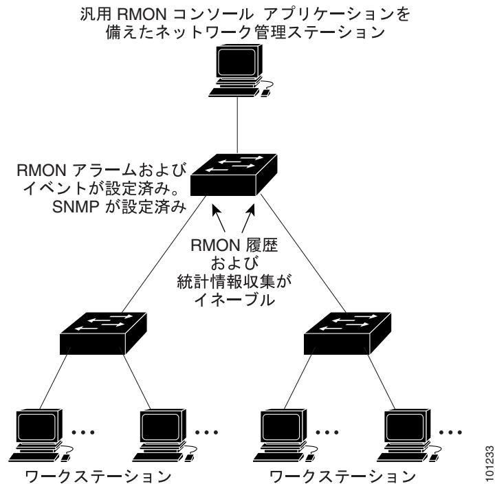
図 28-1 リモート モニタリングの例
