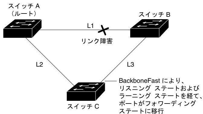
図 19-6 間接リンク障害発生後の BackboneFast の例
