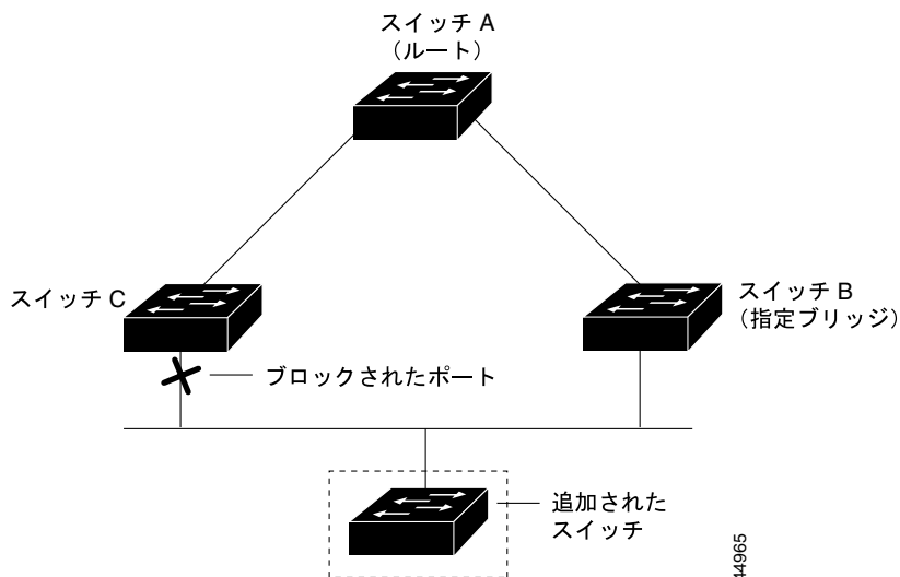
図 19-7 メディア共有型トポロジにおけるスイッチの追加
