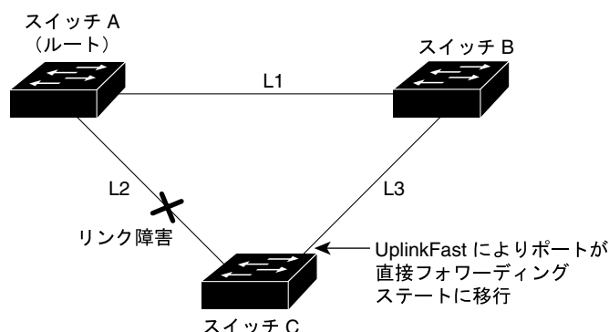
図 19-4 直接リンク障害発生後の UplinkFast の例
