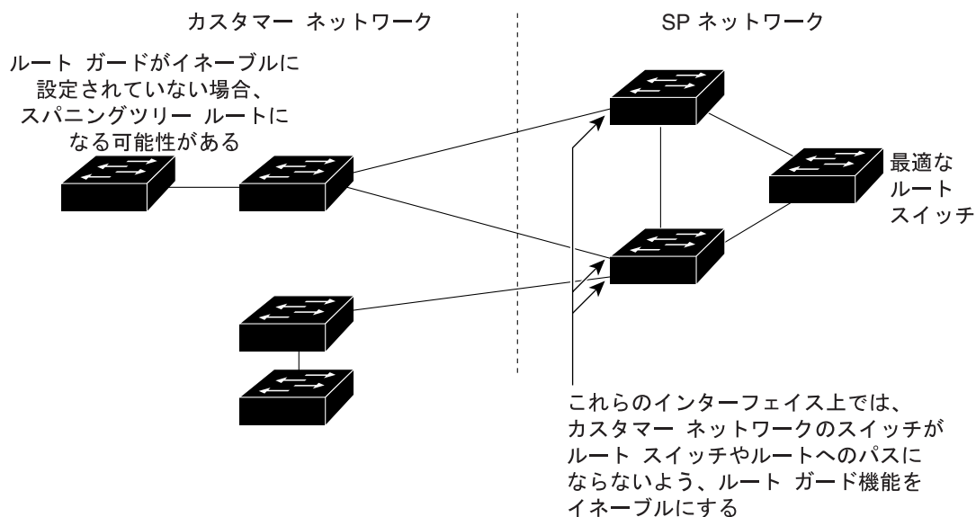
図 19-8 サービス プロバイダー ネットワークのルート ガード
