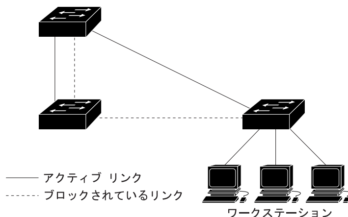
図 17-3 スパニングツリーおよび冗長接続
