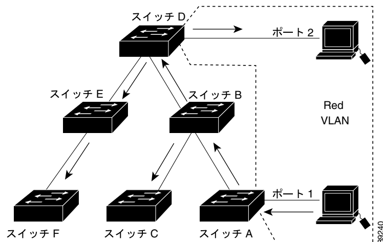
図 13-1 VTP ブルーニングを使用しない場合のフラディング ट्रフィック
