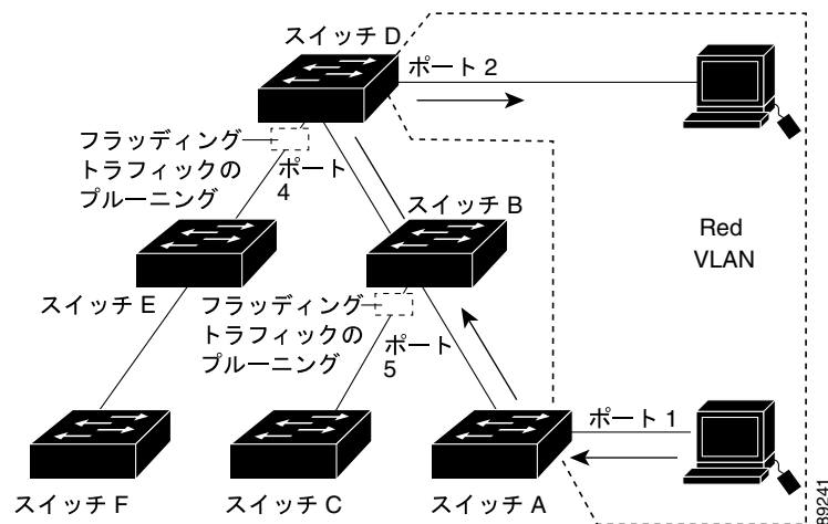
図 13-2 VTP ブルーニングによるフラディング ट्रフィックの最適化
